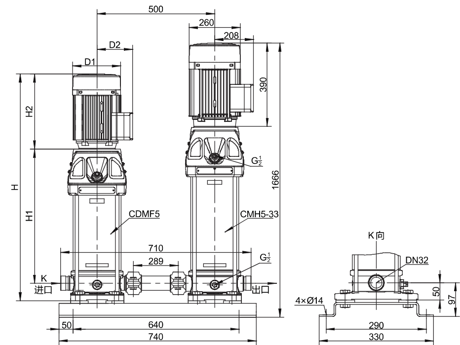
CDMF5+CMH5-33 安装尺寸图
