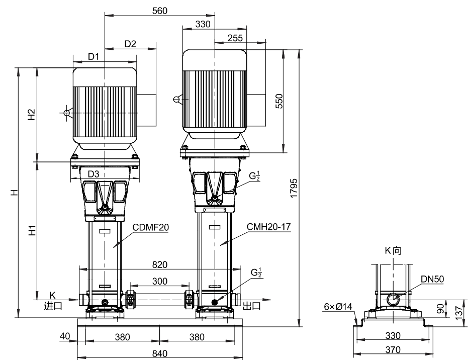
CDMF20+CMH20-17 安装尺寸图
