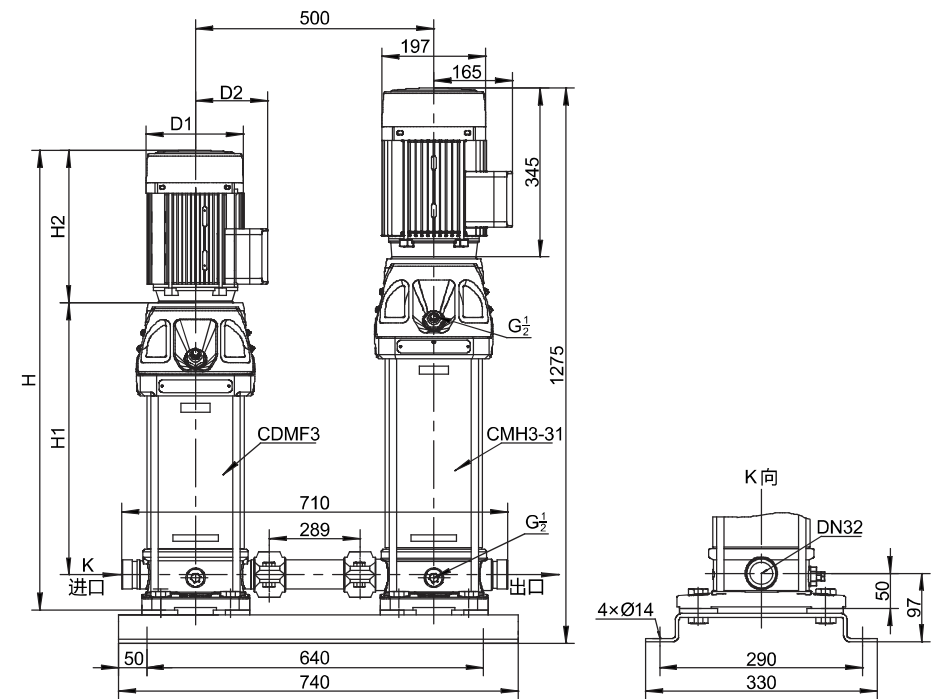
CDMF3+CMH3-31 安装尺寸图
