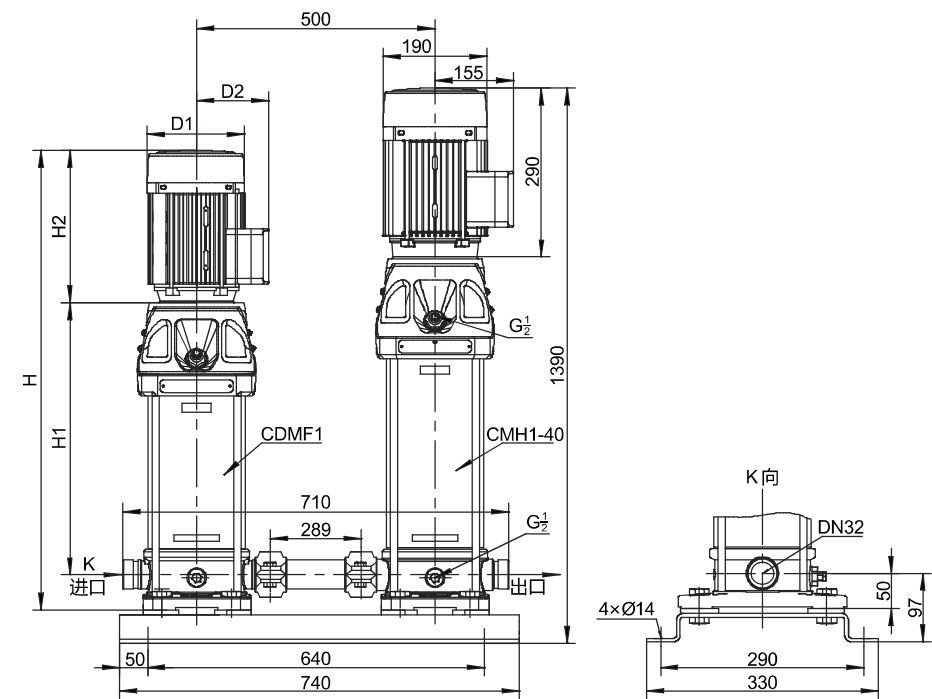
CDMF1+CMH1-40 安装尺寸图
