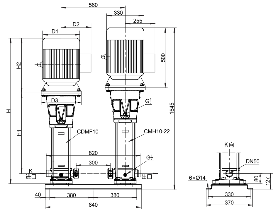
CDMF10+CMH10-22 安装尺寸图
