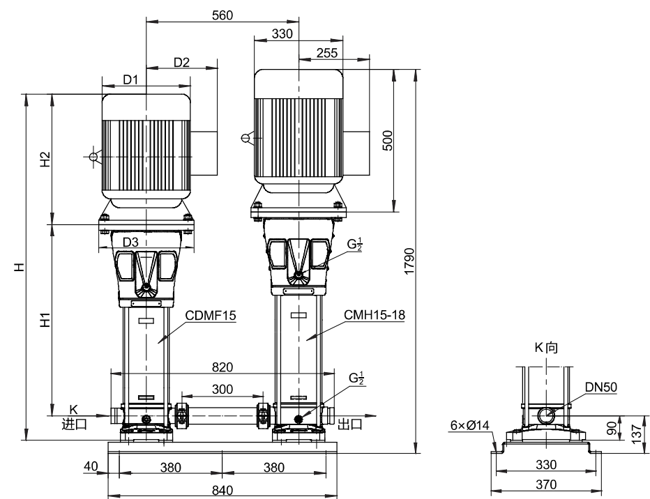
CDMF15+CMH15-18 安装尺寸图
