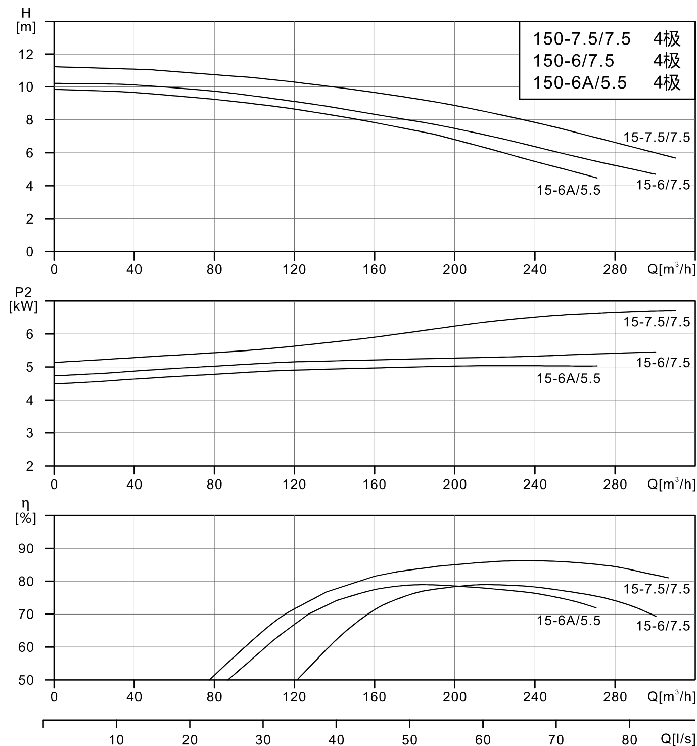
WLT/WLTS/WLTSF(50Hz)性能曲线
