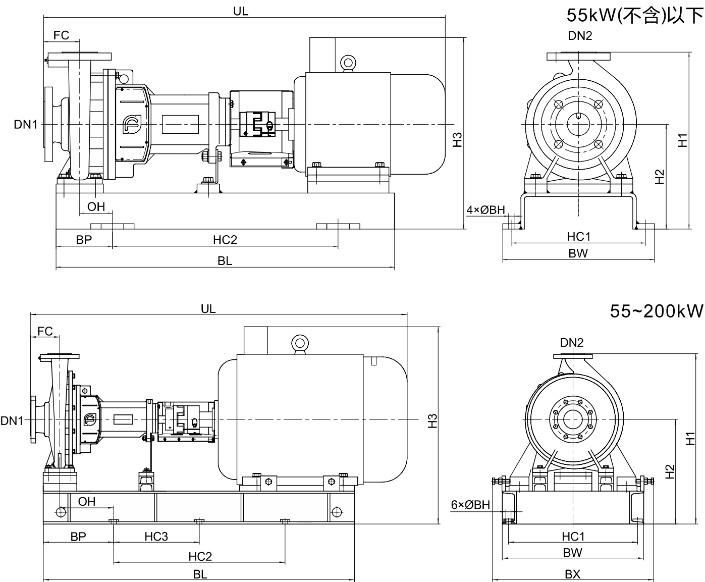
NISO*G,NISO*(Q)泵组外形尺寸表
