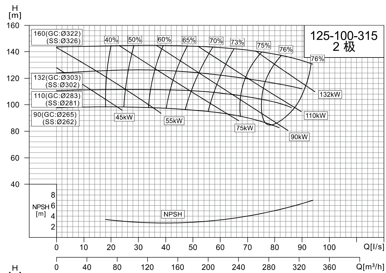
NISO,NIS,NISF125-100-315/50-32-160
