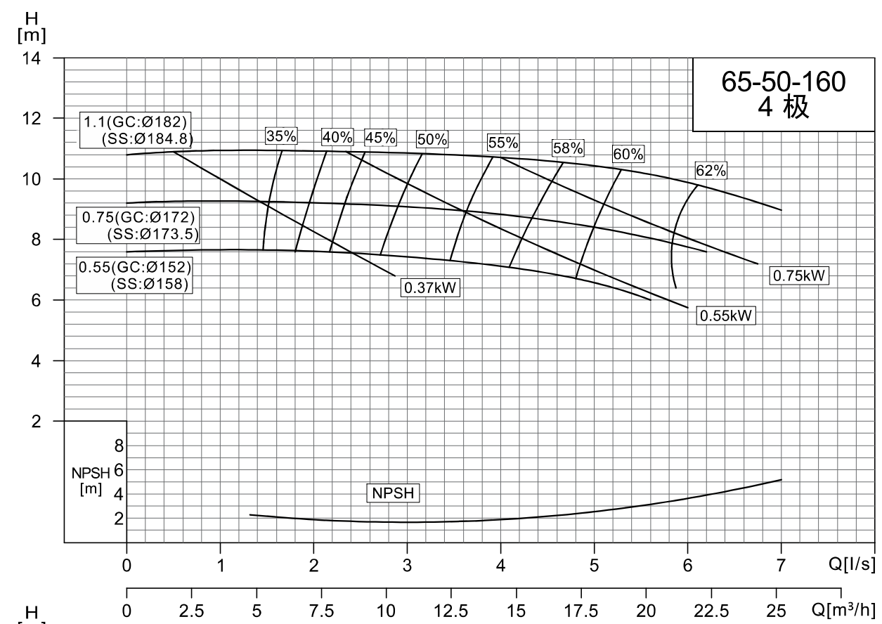
NISO,NIS,NISF65-50-160/80-50-200
