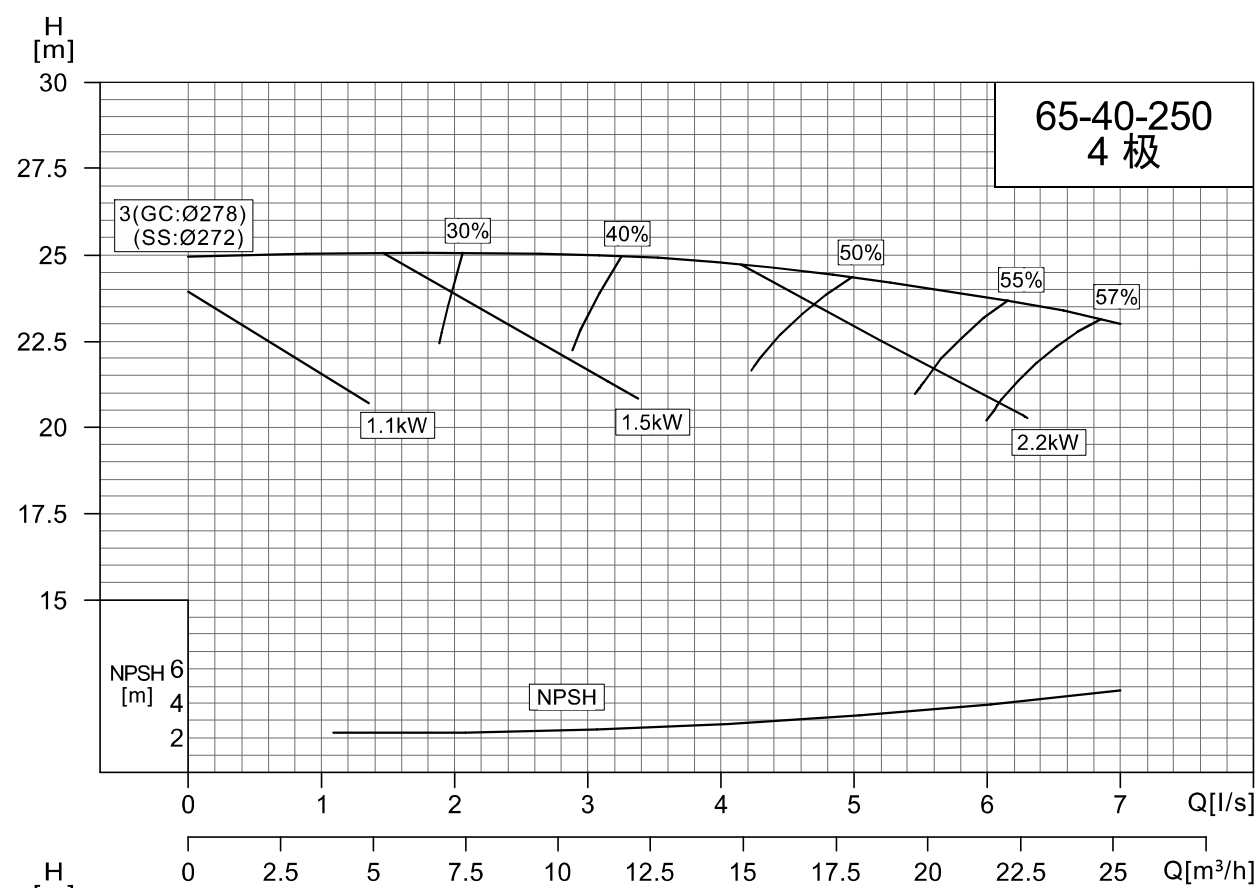
NISO,NIS,NISF65-40-250/65-40-315
