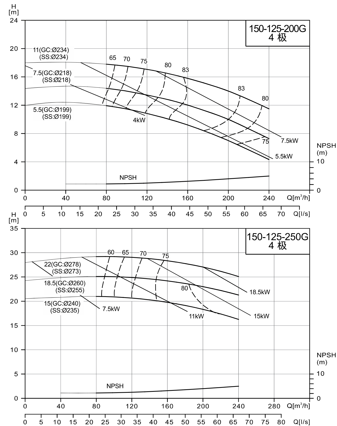
NISO/NIS/NISF150-125-200G/150-125-250G
