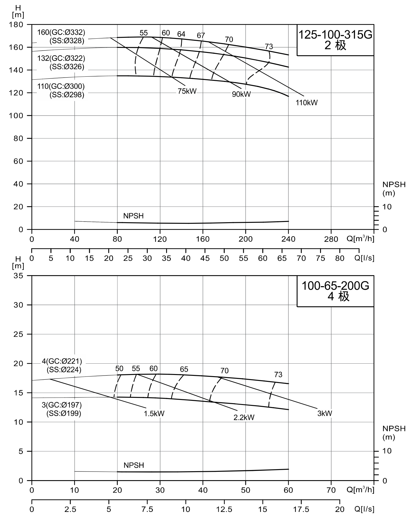
NISO/NIS/NISF125-100-315G/100-65-200G
