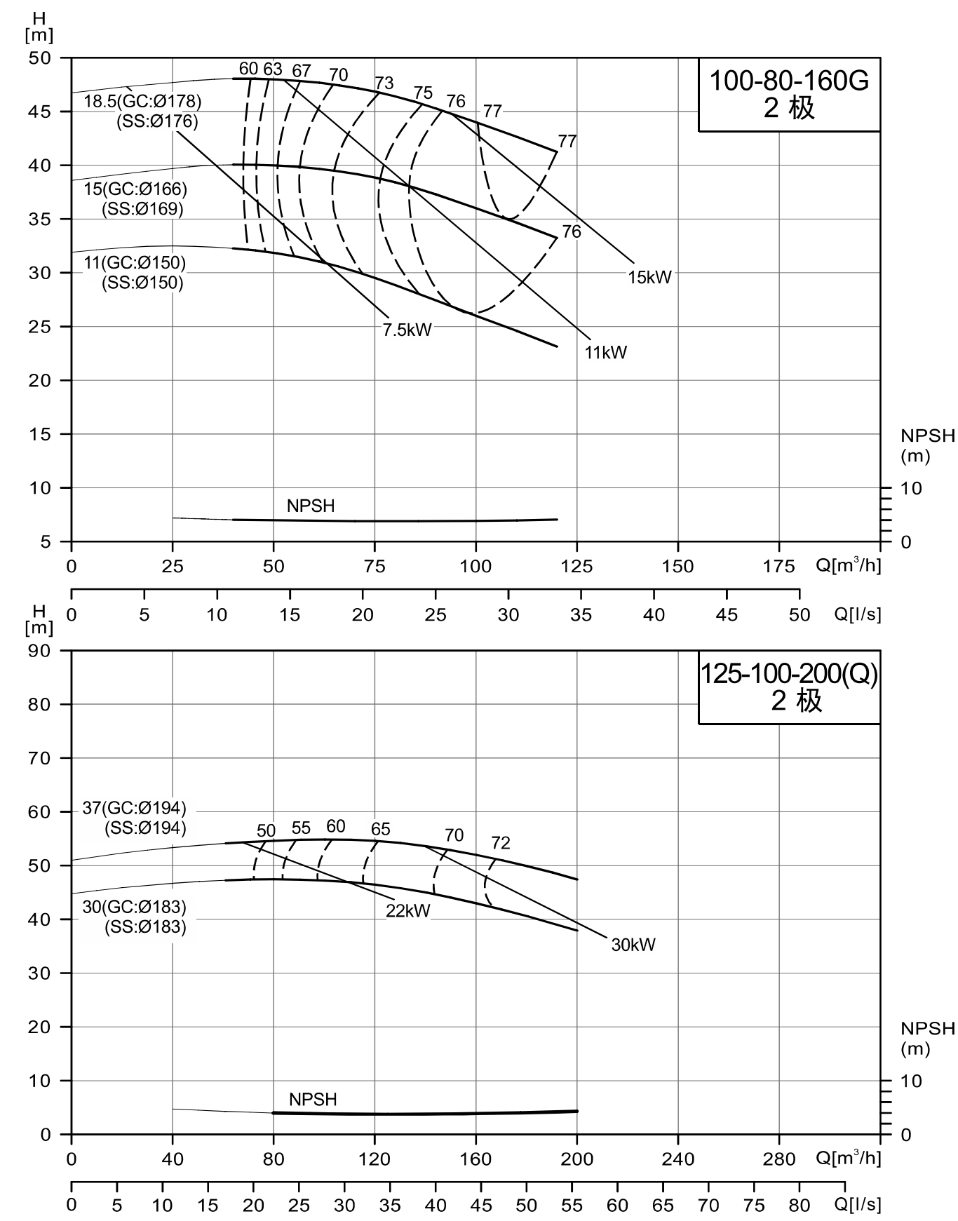
NISO/NIS/NISF100-80-160G/125-100-200(Q)
