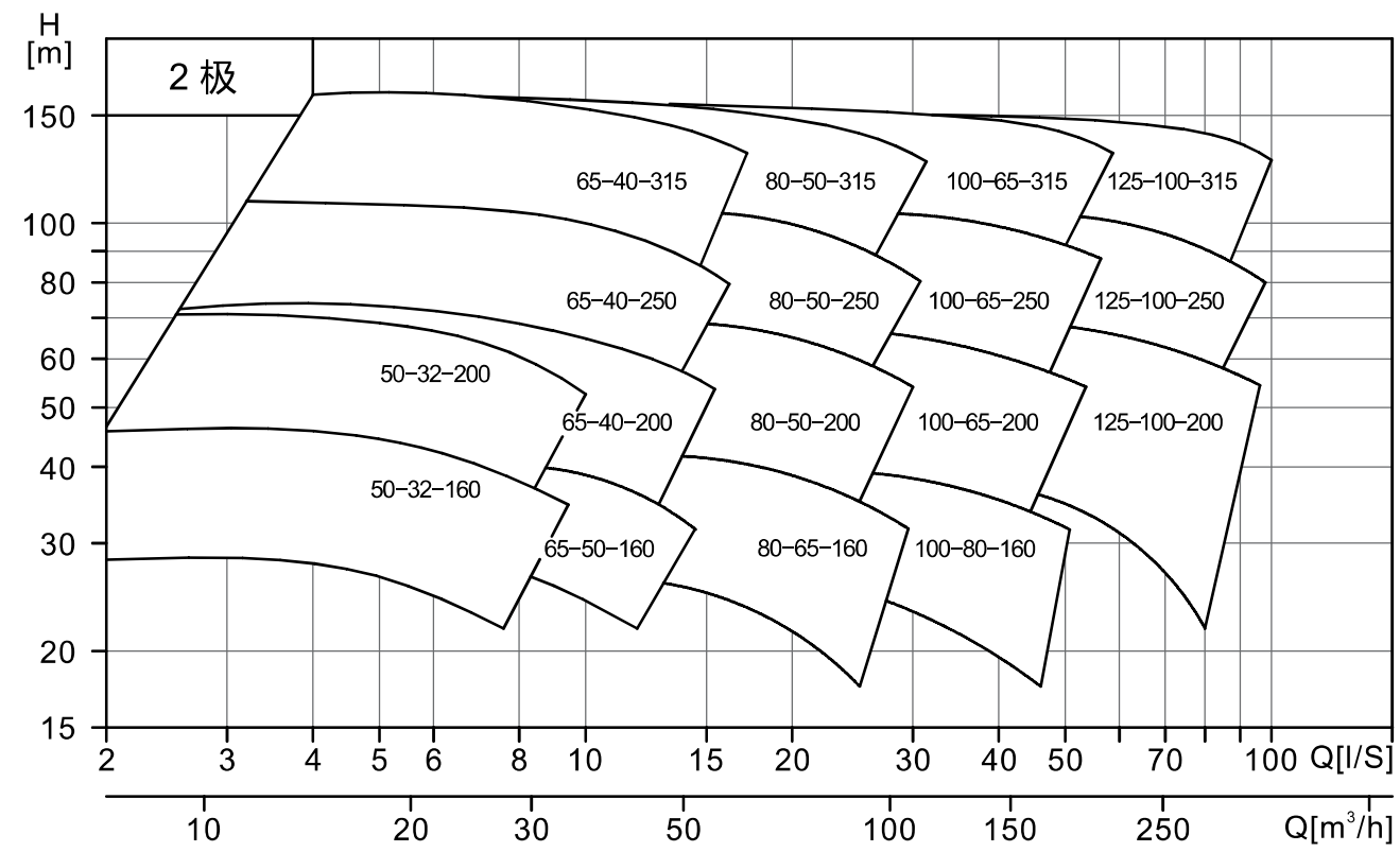
NISO,NIS,NISF型谱图
