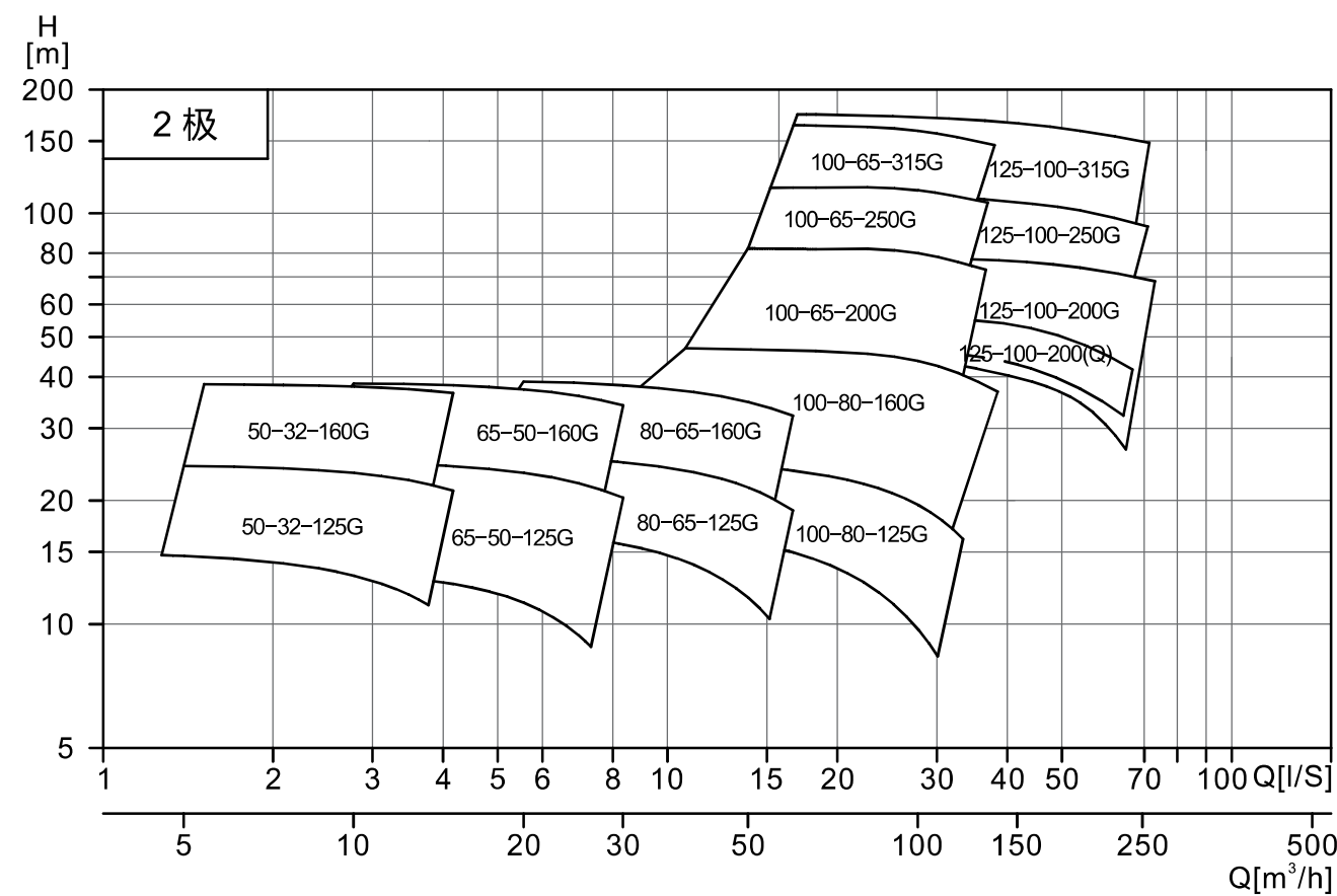
NISO/NIS/NISF*G,NISO/NIS/NISF*(Q)型谱图
