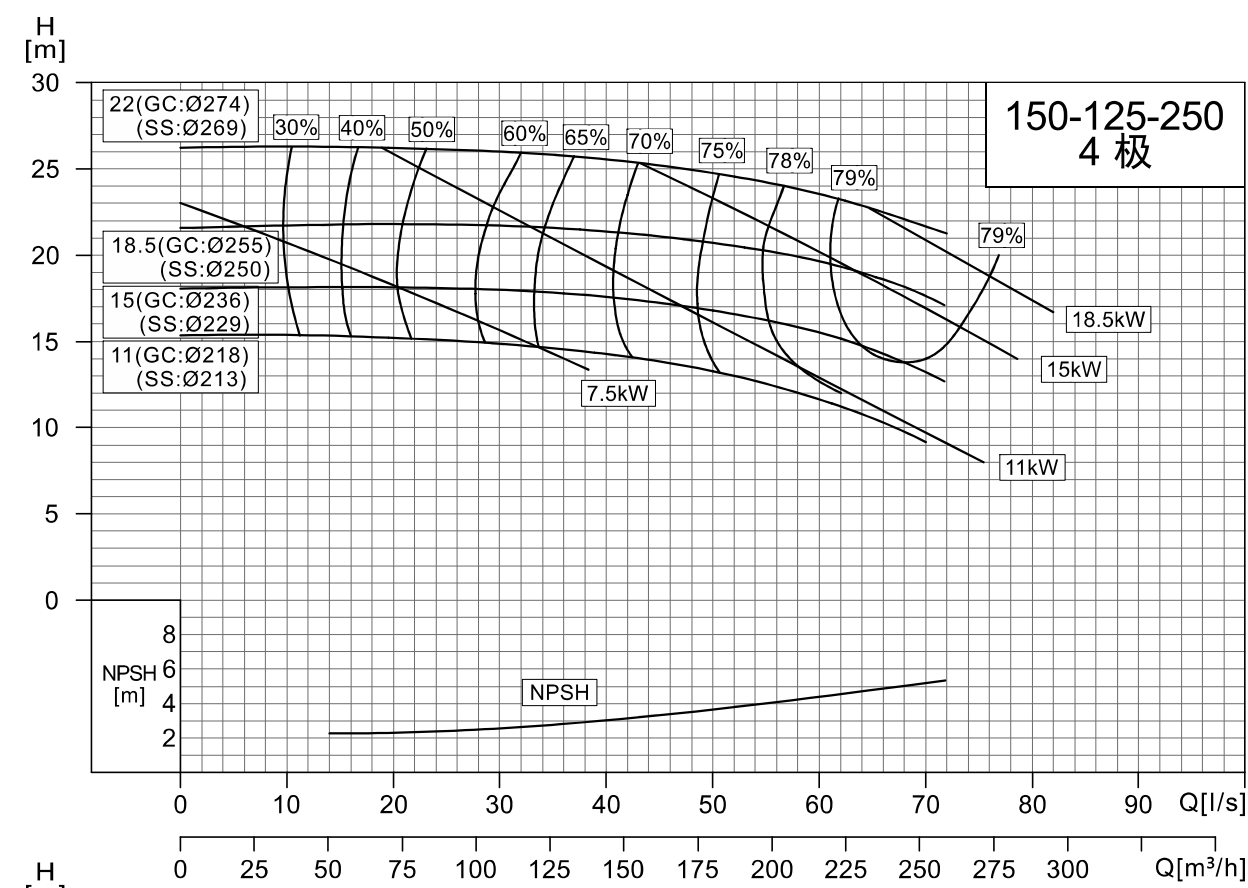
NISO,NIS,NISF150-125-250/150-125-315
