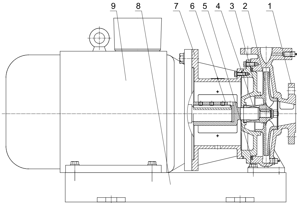
NIS,NISF截面图
