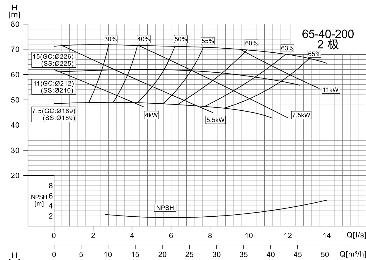
NISO,NIS,NISF65-40-200/65-40-250
