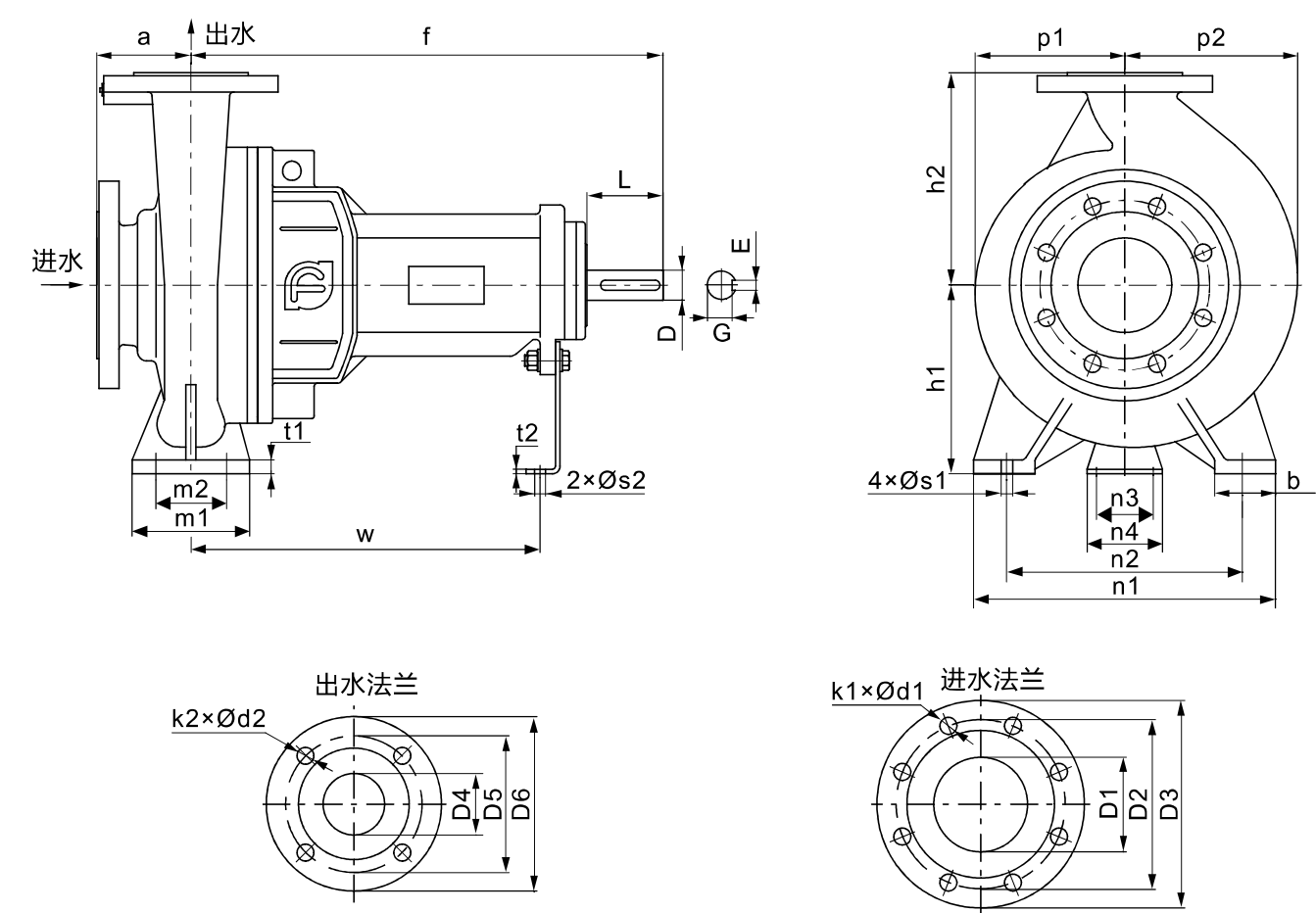
NISO*G,NISO*(Q)泵外形尺寸图
