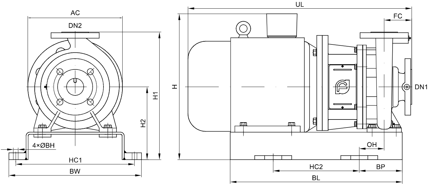
NIS/NISF*G,NIS/NISF*(Q)泵外形尺寸图
