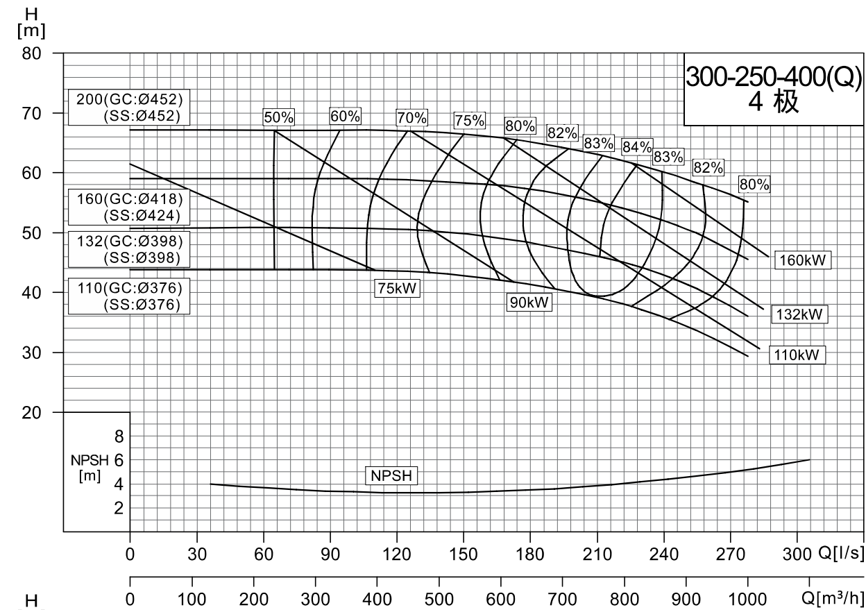
NISO,NIS,NISF300-250-400(Q)/300-250-400
