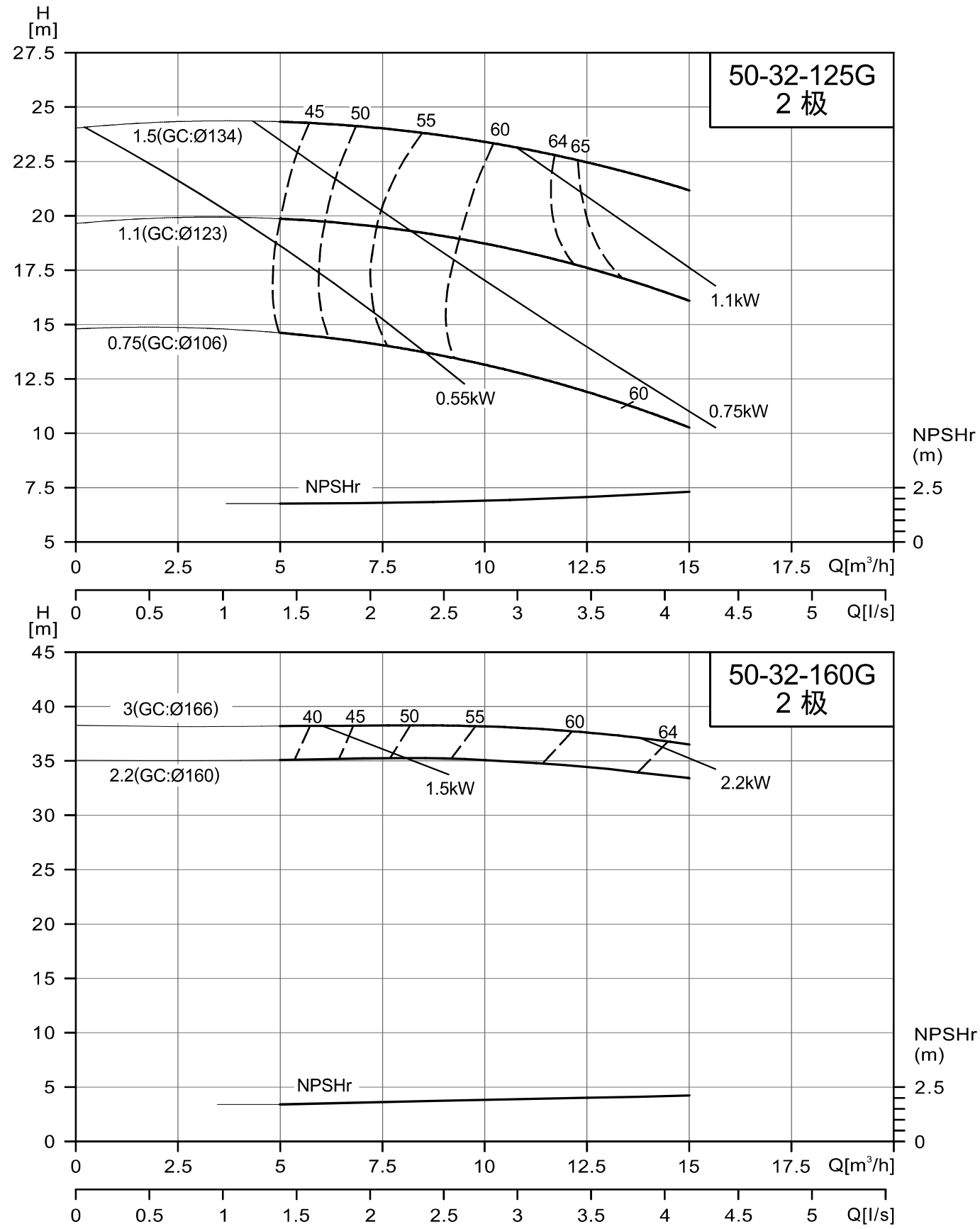
NISO/NIS/NISF50-32-125G/50-32-160G
