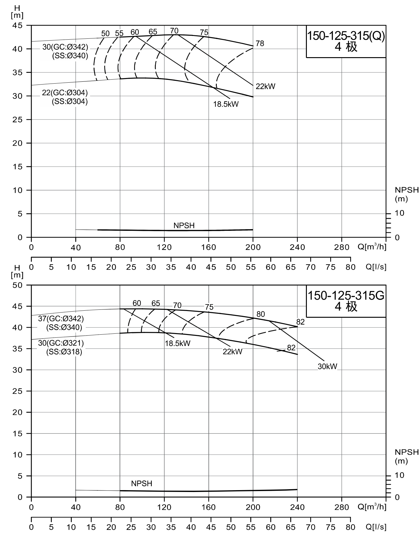
NISO/NIS/NISF150-125-315(Q)/150-125-315G
