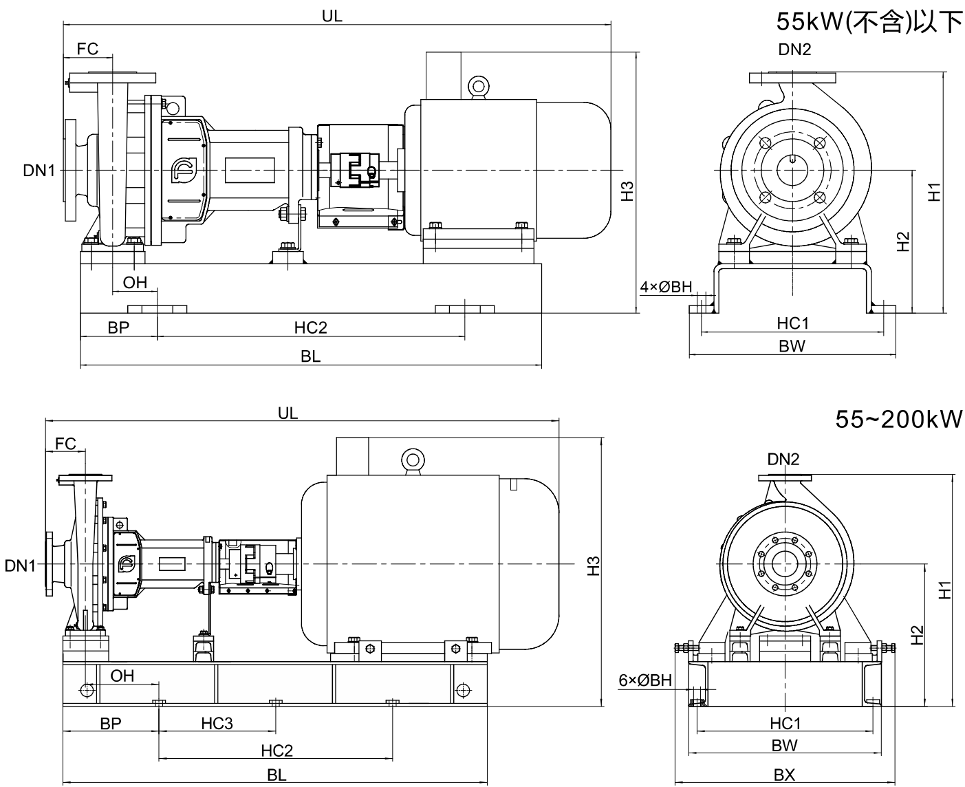
NISO泵组外形尺寸表
