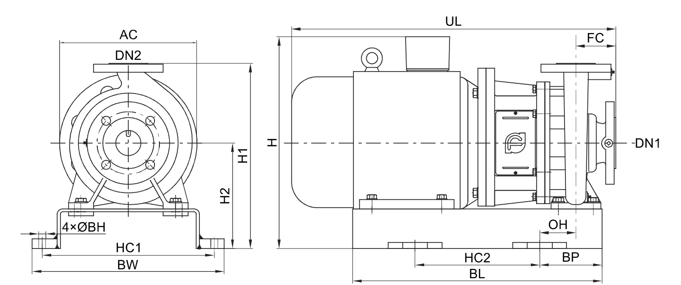
NIS,NISF泵外形尺寸图
