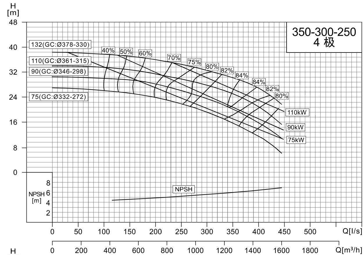
NISO,NIS,NISF350-300-250/350-300-315
