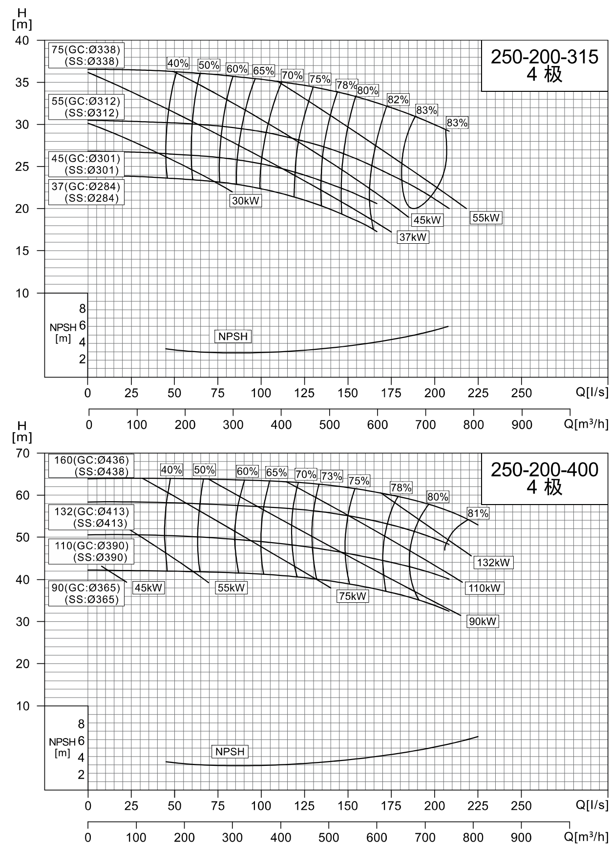
NISO,NIS,NISF250-200-315/250-200-400
