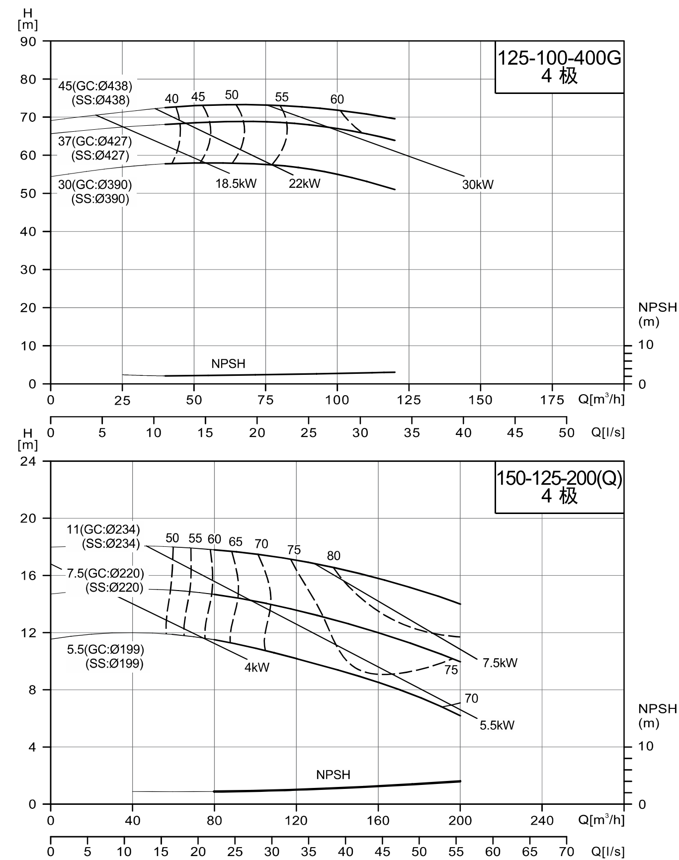
NISO/NIS/NISF125-100-400G/150-125-200(Q)
