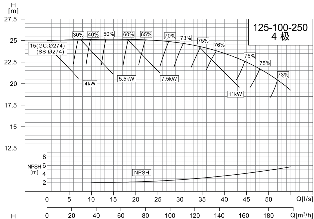
NISO,NIS,NISF125-100-250/125-100-315
