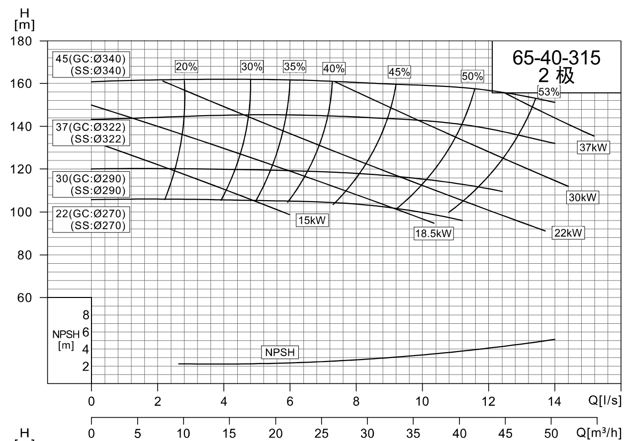
NISO,NIS,NISF65-40-315/65-50-160
