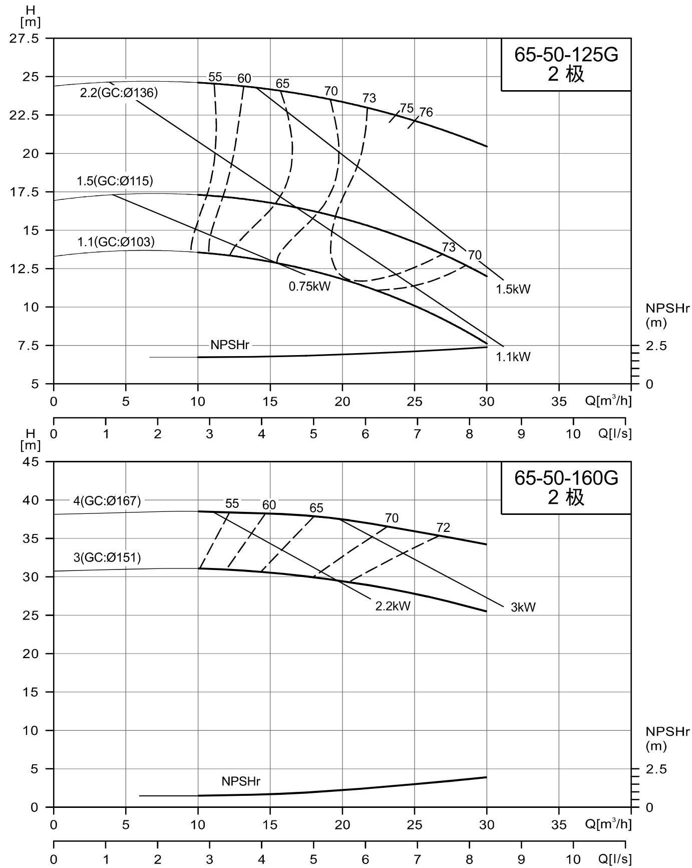
NISO/NIS/NISF65-50-125G/65-50-160G
