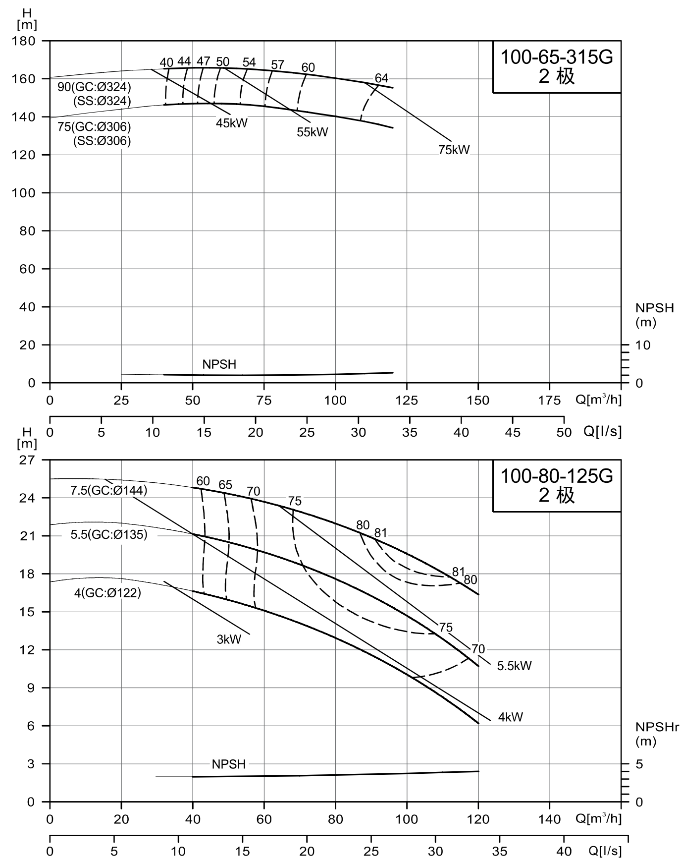
NISO/NIS/NISF100-65-315G/100-80-125G
