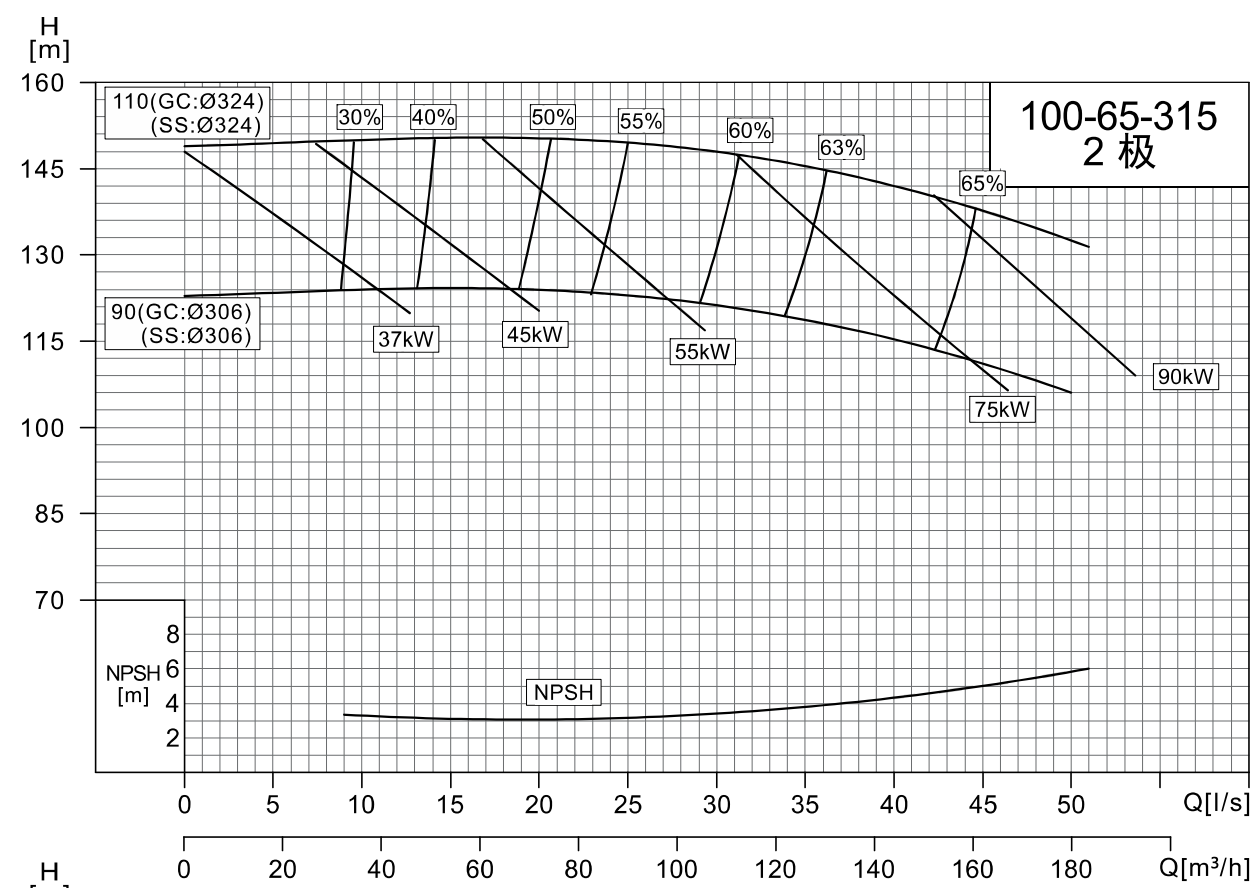
NISO,NIS,NISF100-65-315/100-80-160
