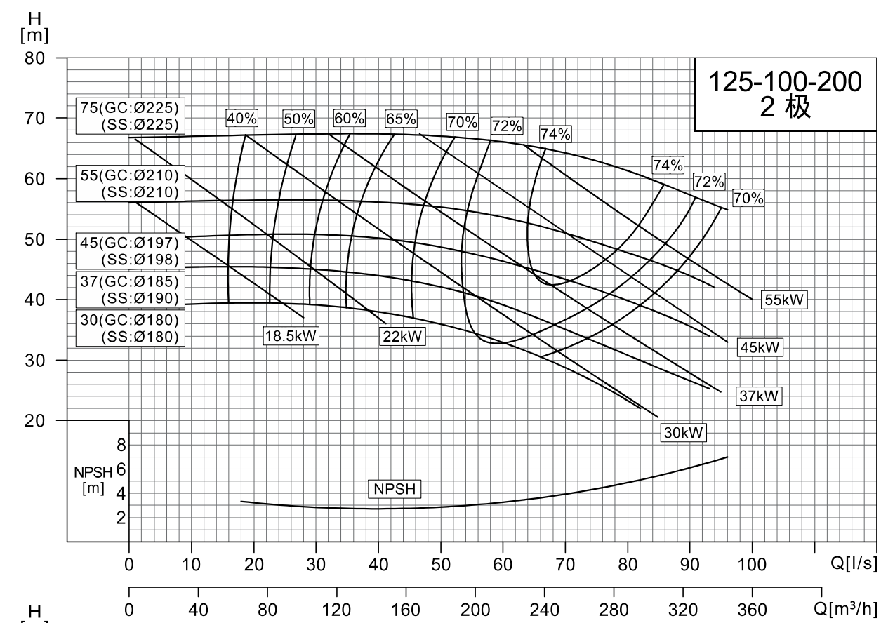
NISO,NIS,NISF125-100-200/125-100-250
