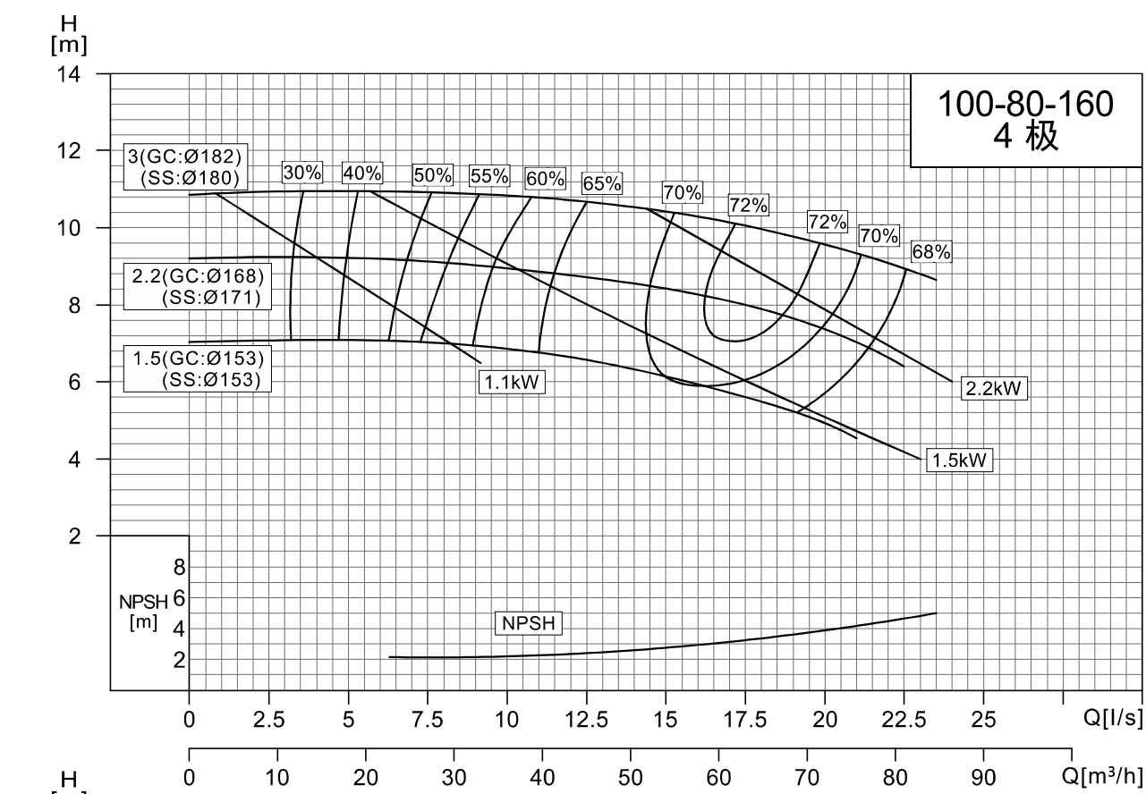
NISO,NIS,NISF100-80-160/125-100-200
