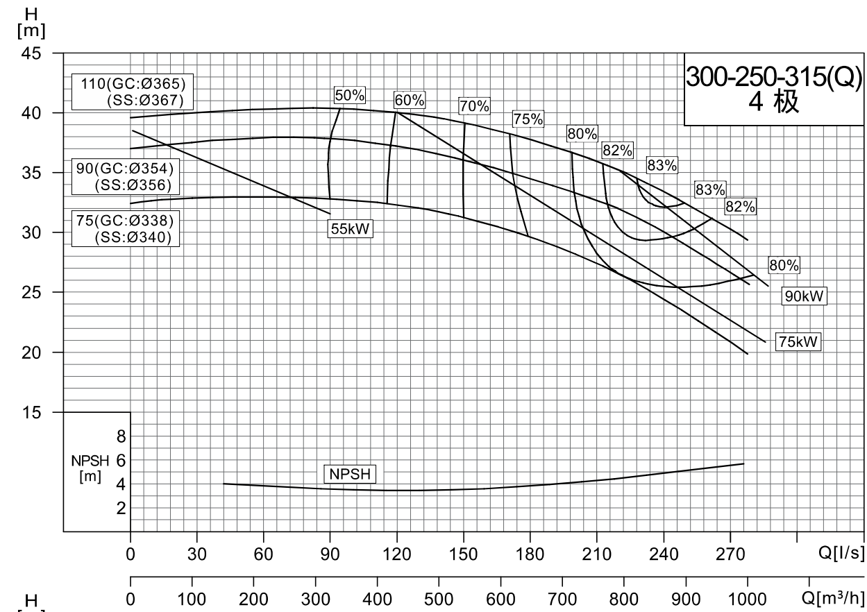
NISO,NIS,NISF300-250-315(Q)/300-250-315
