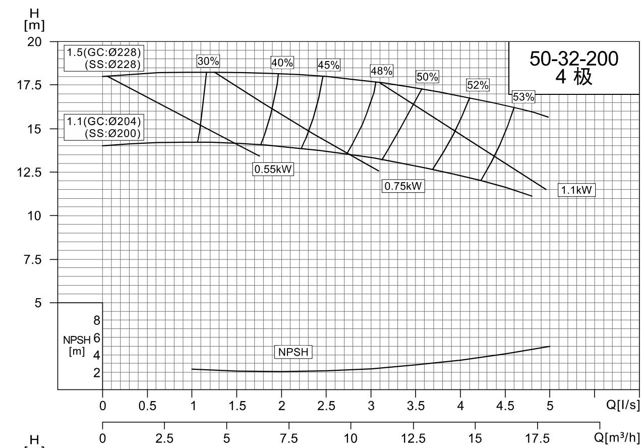
NISO,NIS,NISF50-32-200/65-40-200
