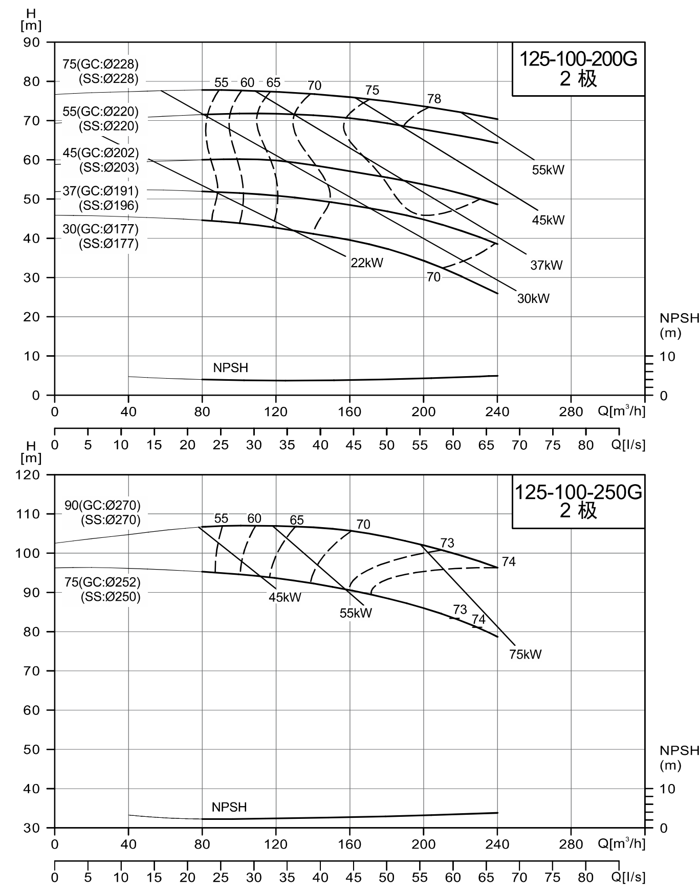
NISO/NIS/NISF125-100-200G/125-100-250G
