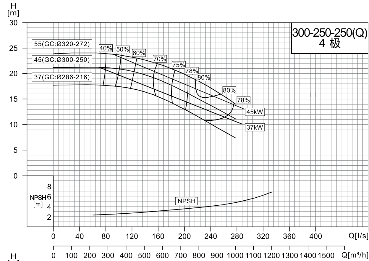
NISO,NIS,NISF300-250-250(Q)/300-250-250
