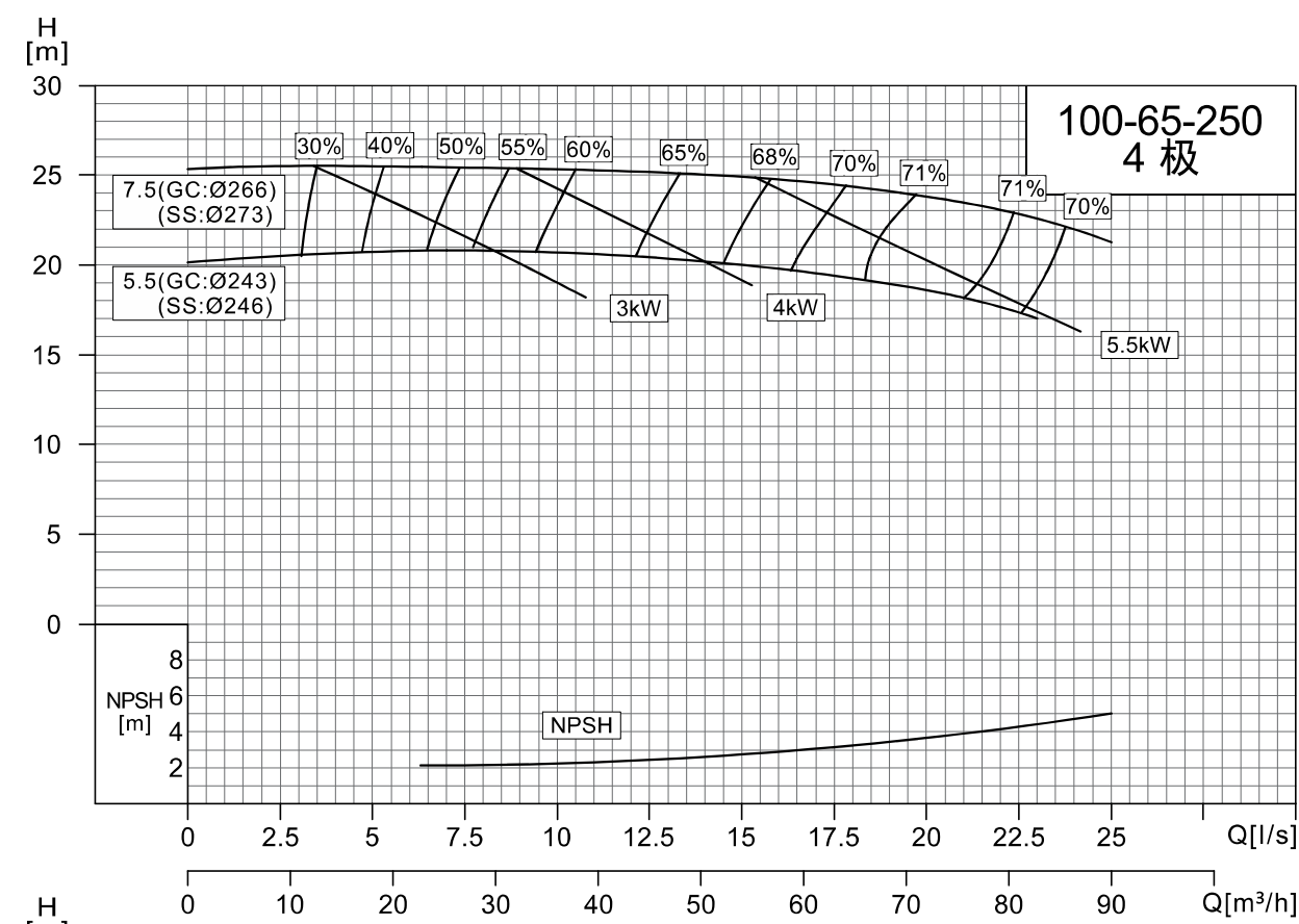
NISO,NIS,NISF100-65-250/100-65-315
