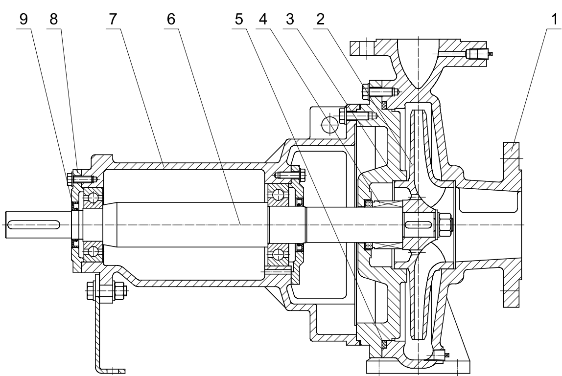
NISO截面图
