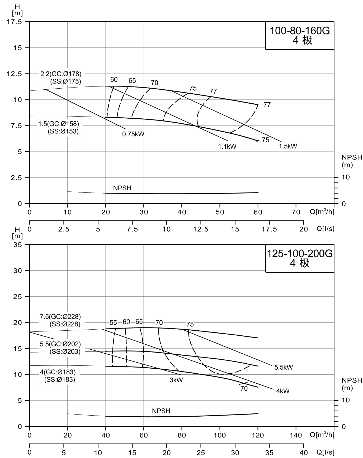
NISO/NIS/NISF100-80-160G/125-100-200G
