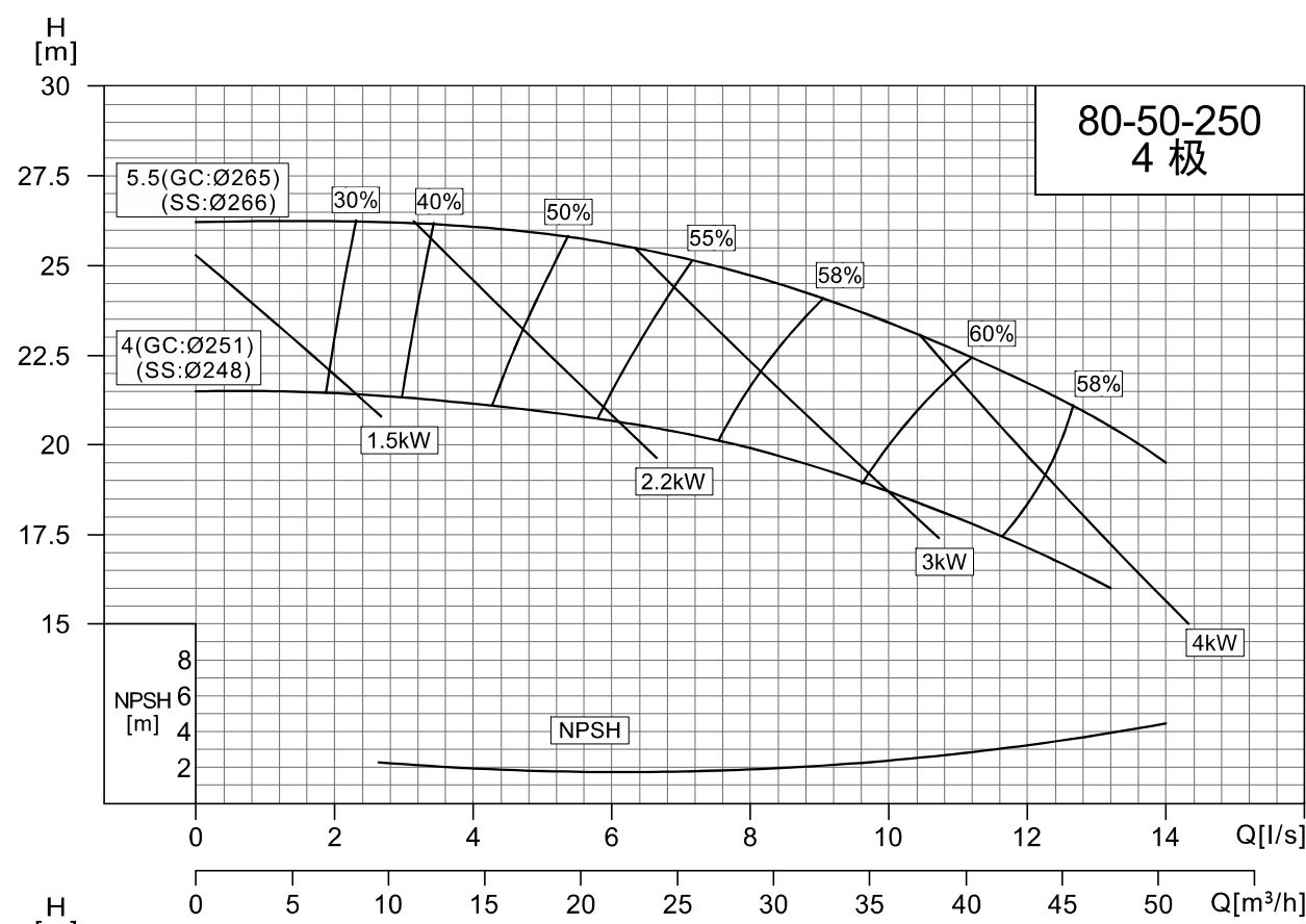
NISO,NIS,NISF80-50-250/80-50-315
