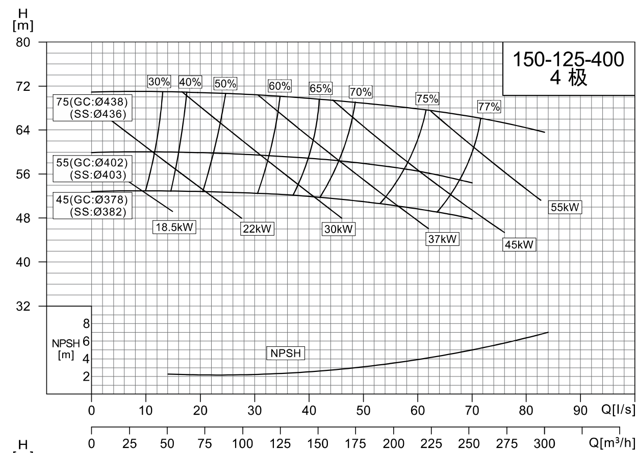
NISO,NIS,NISF150-125-400/200-150-315
