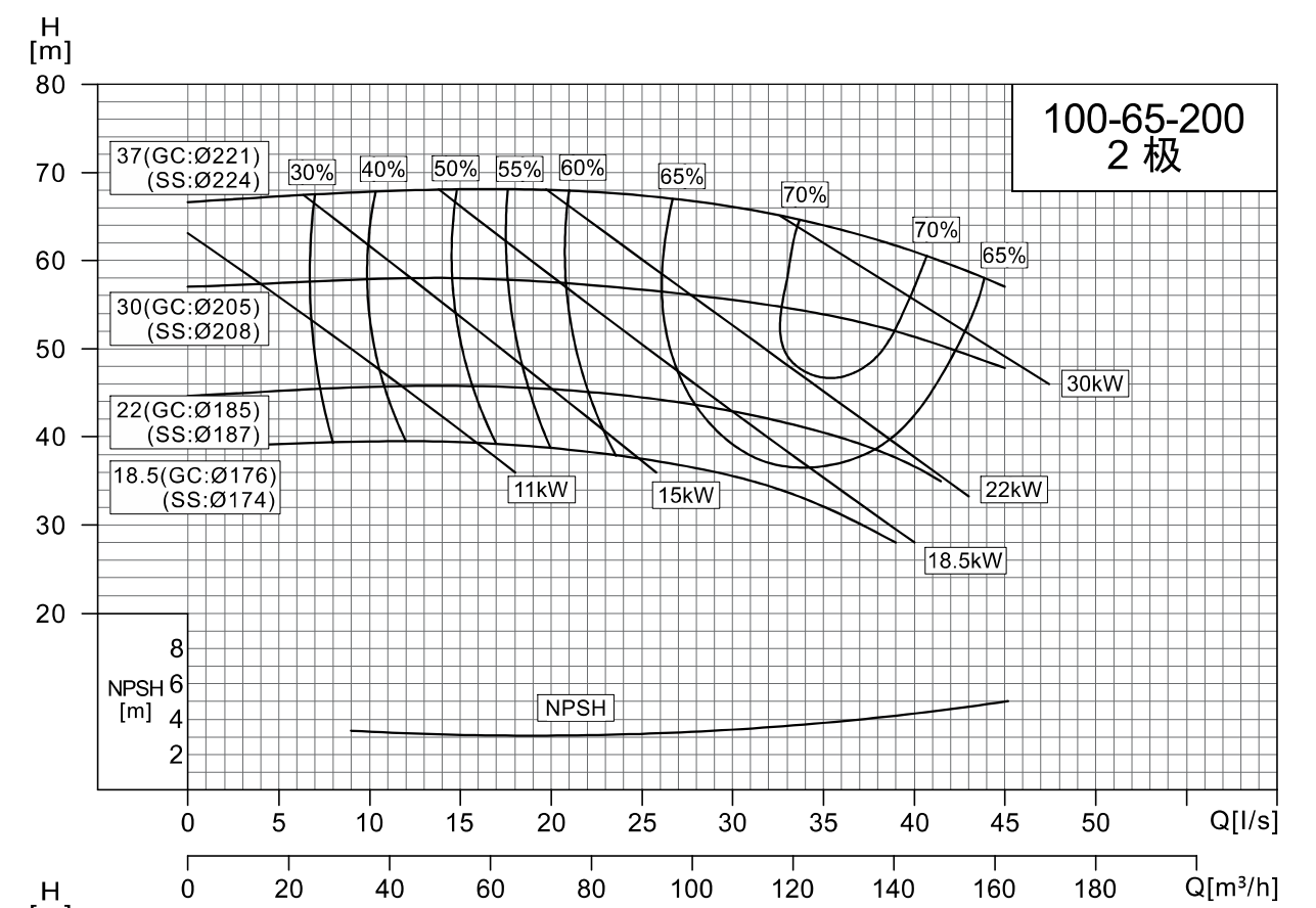
NISO,NIS,NISF100-65-200/100-65-250
