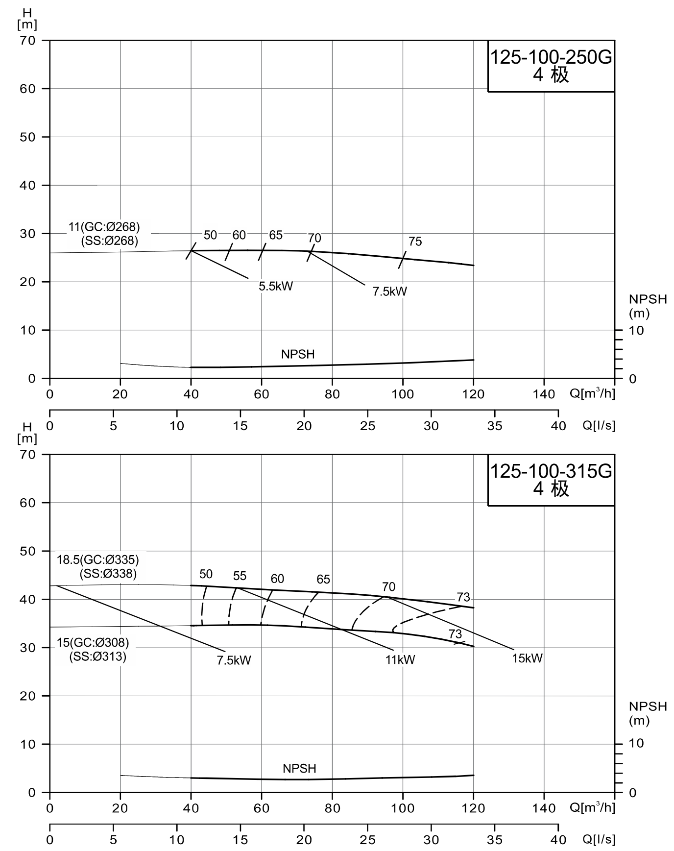
NISO/NIS/NISF125-100-250G/125-100-315G
