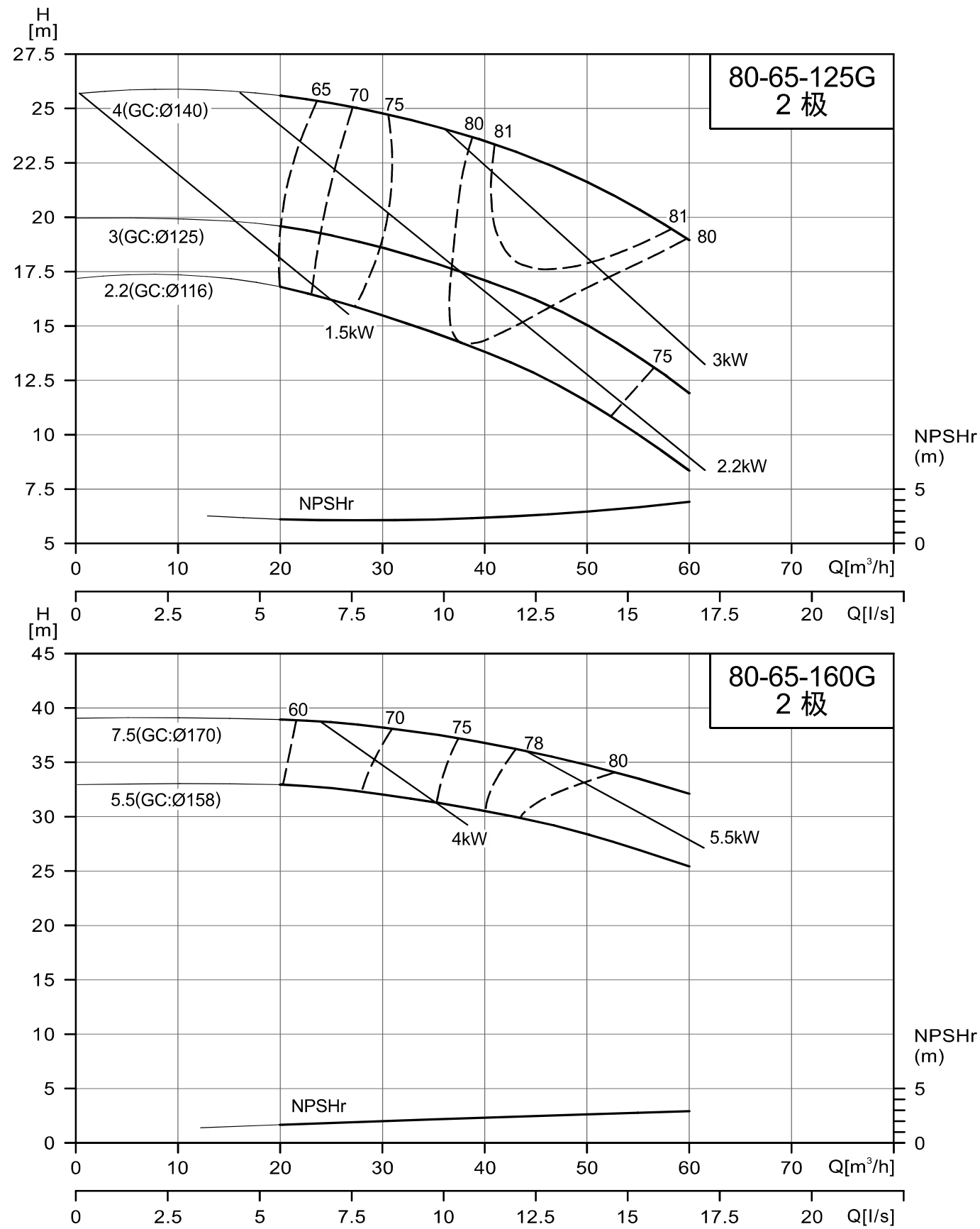
NISO/NIS/NISF80-65-125G/80-65-160G
