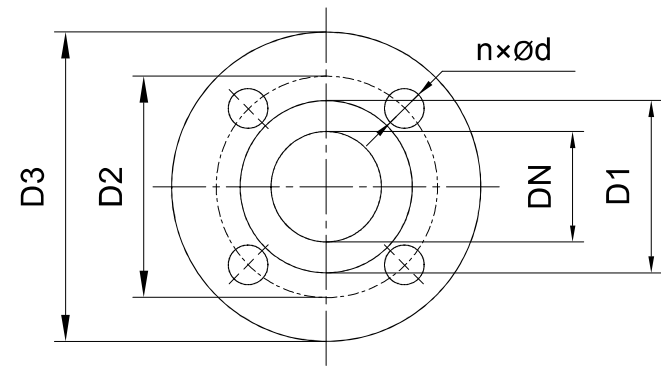
NIS/NISF*G,NIS/NISF*(Q)法兰
