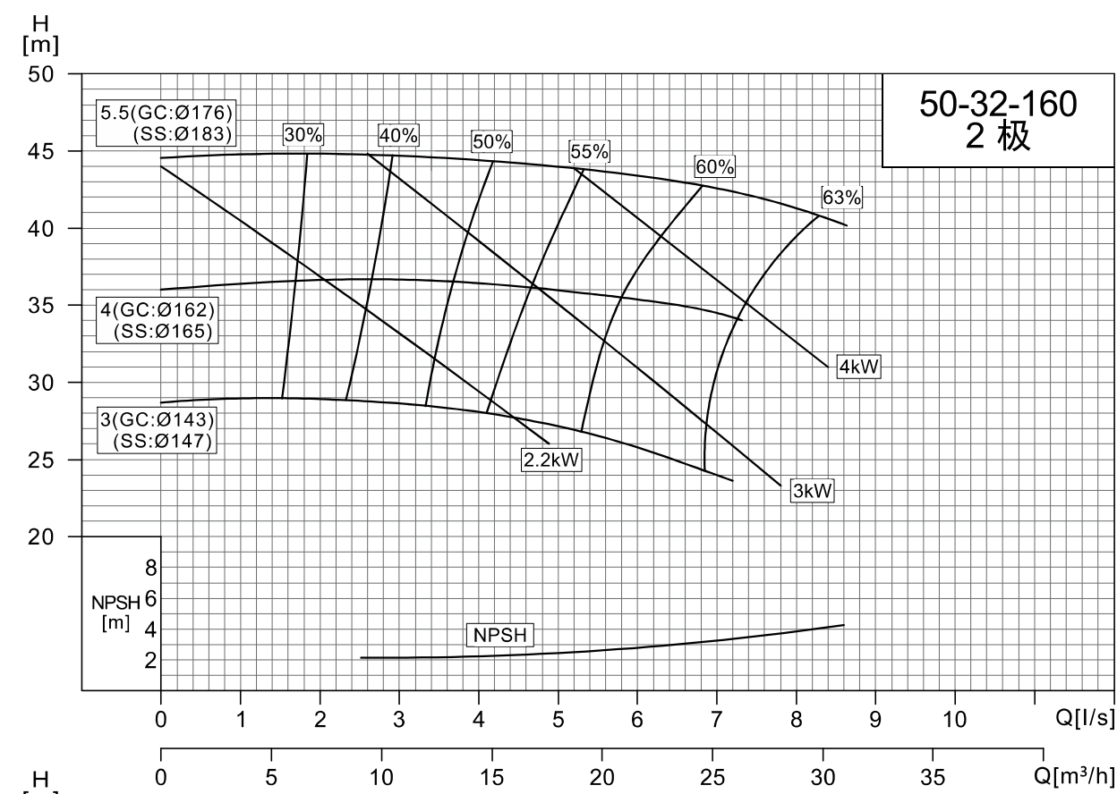
NISO,NIS,NISF50-32-160/50-32-200
