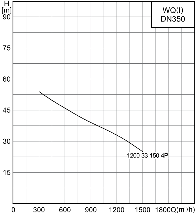
性能曲线
