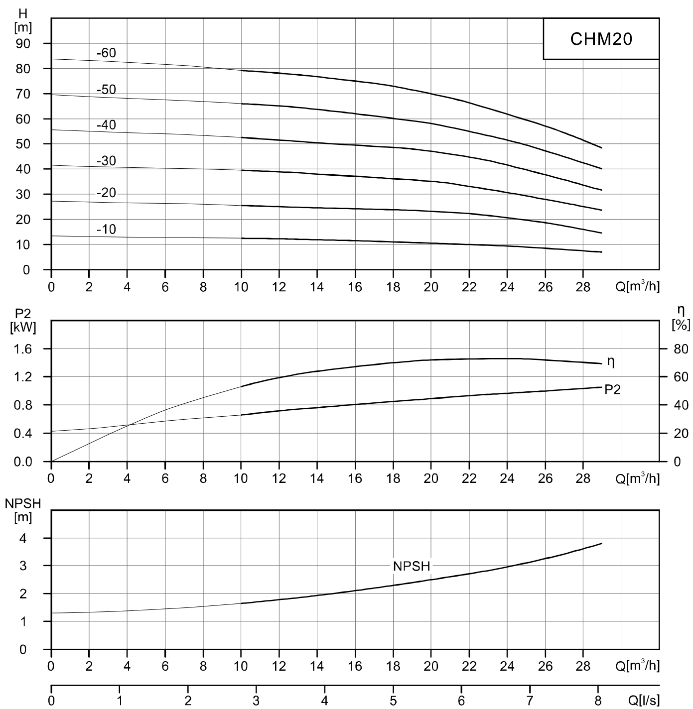
CHM20 性能表
