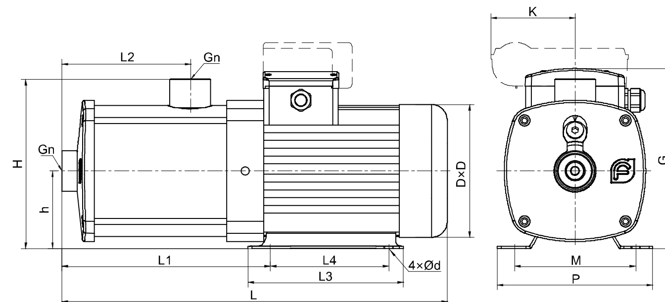
CHM10,15,20,25 尺寸和重量
