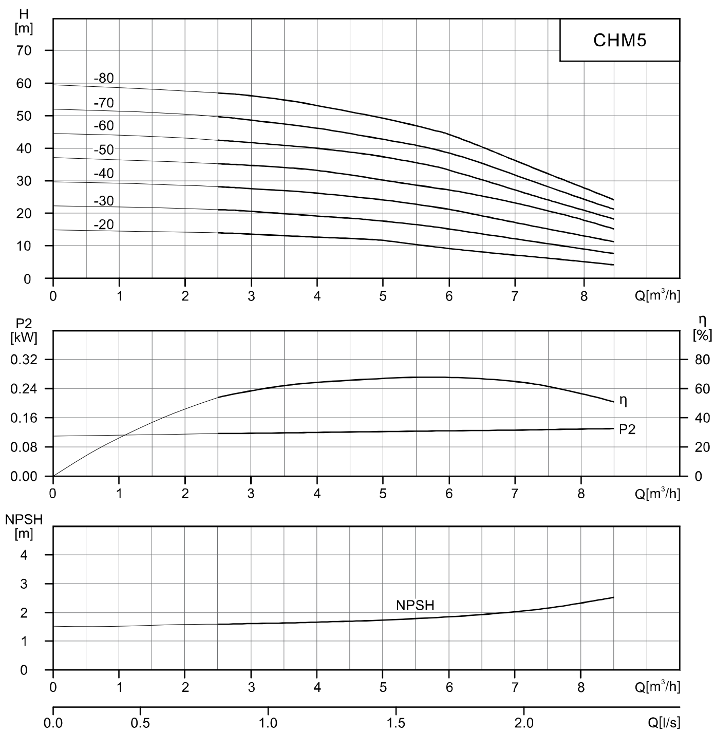
CHM5 性能表
