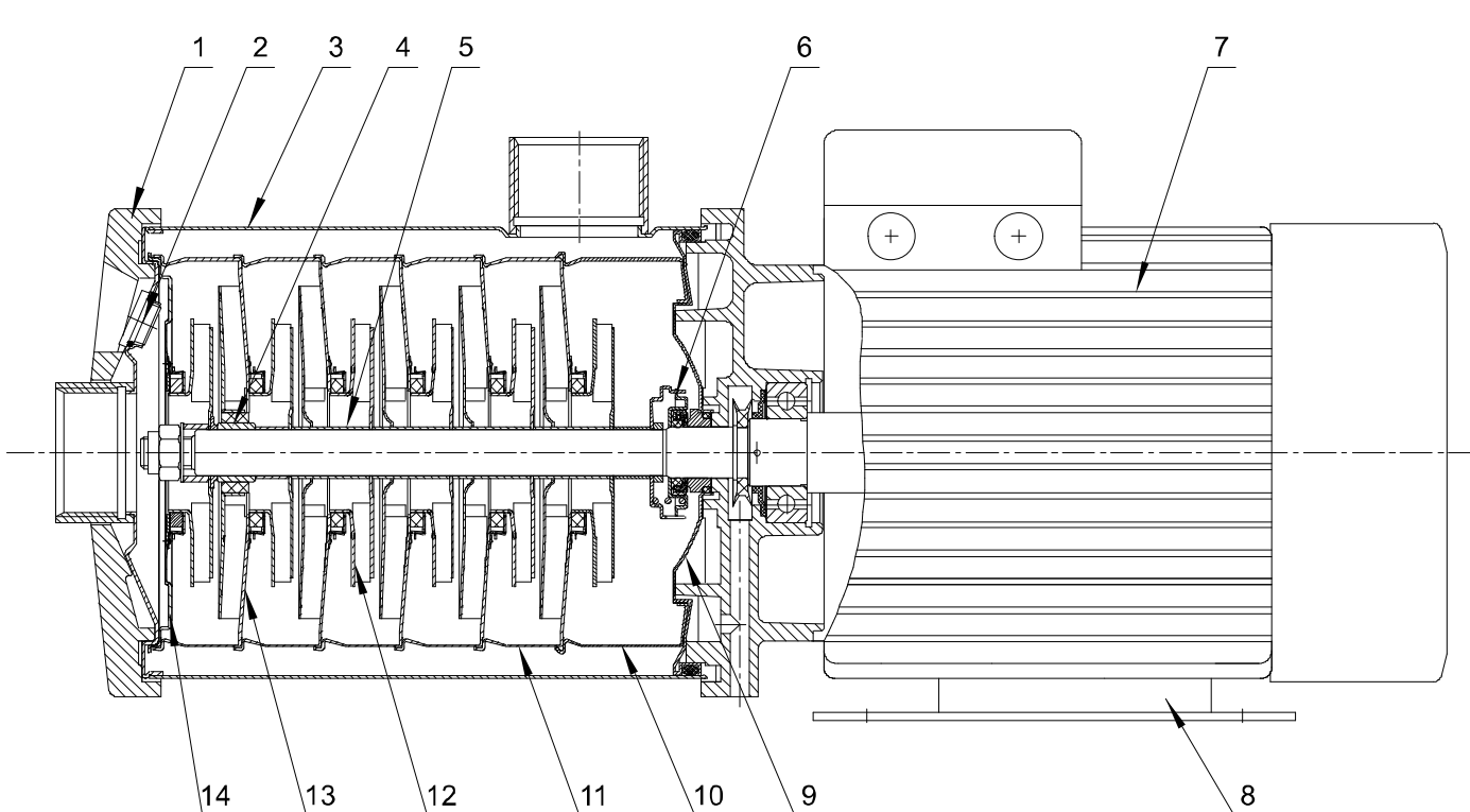
CHM10,25 截面图
