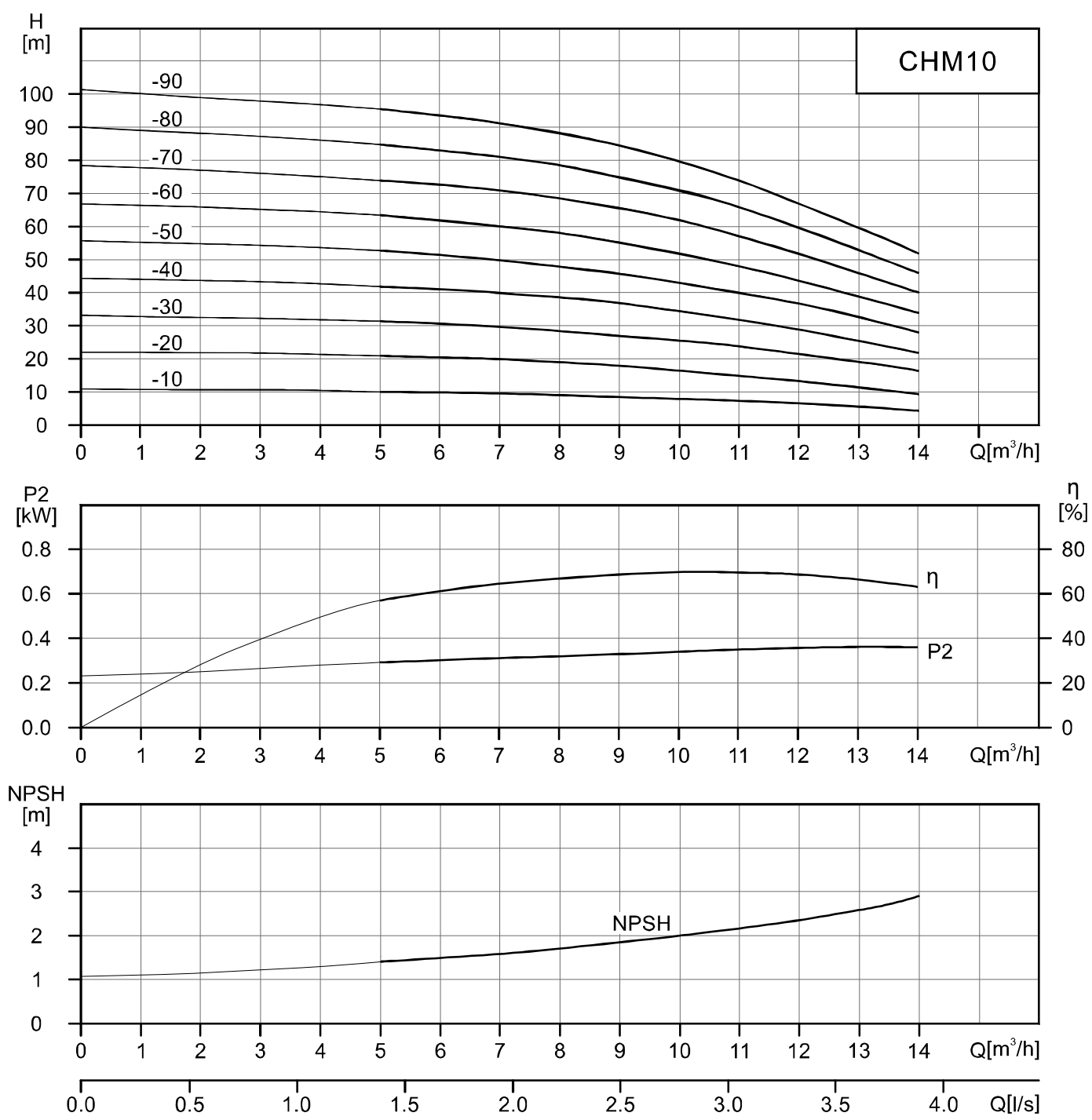
CHM10 性能表
