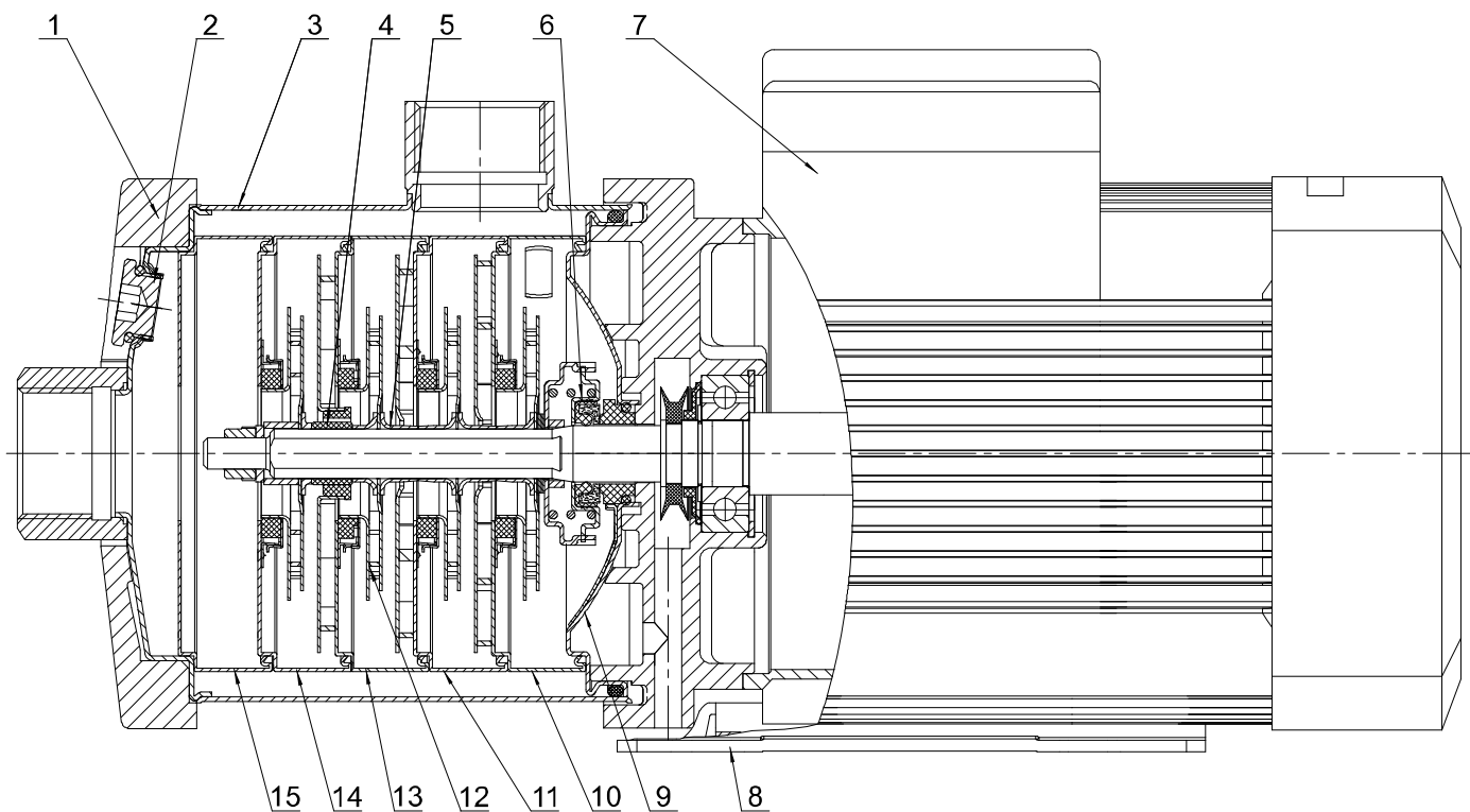
CHM1,3,5 截面图
