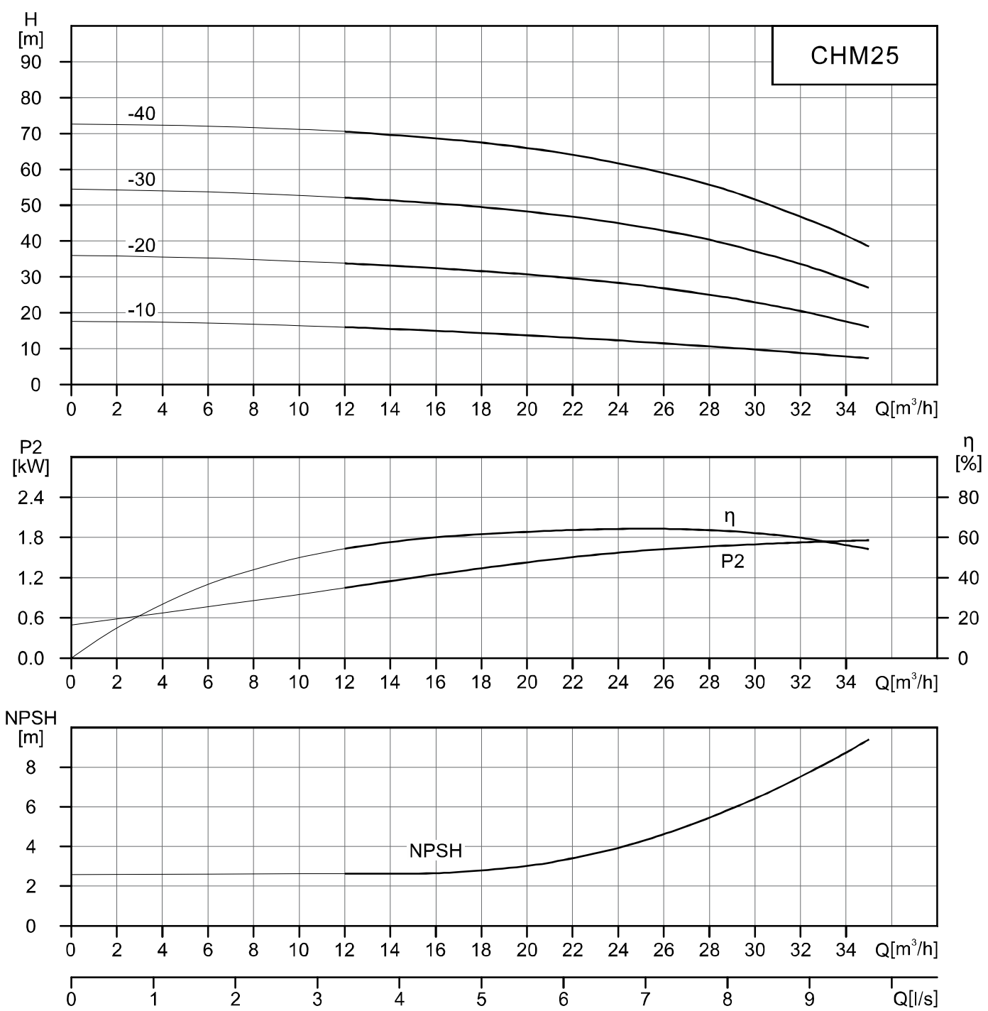
CHM25 性能表
