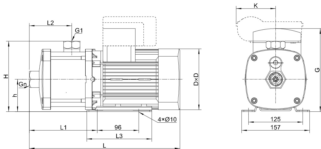
CHM1,3,5 尺寸和重量
