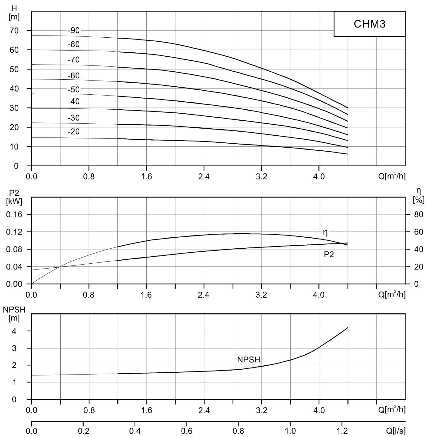
CHM3 性能表
