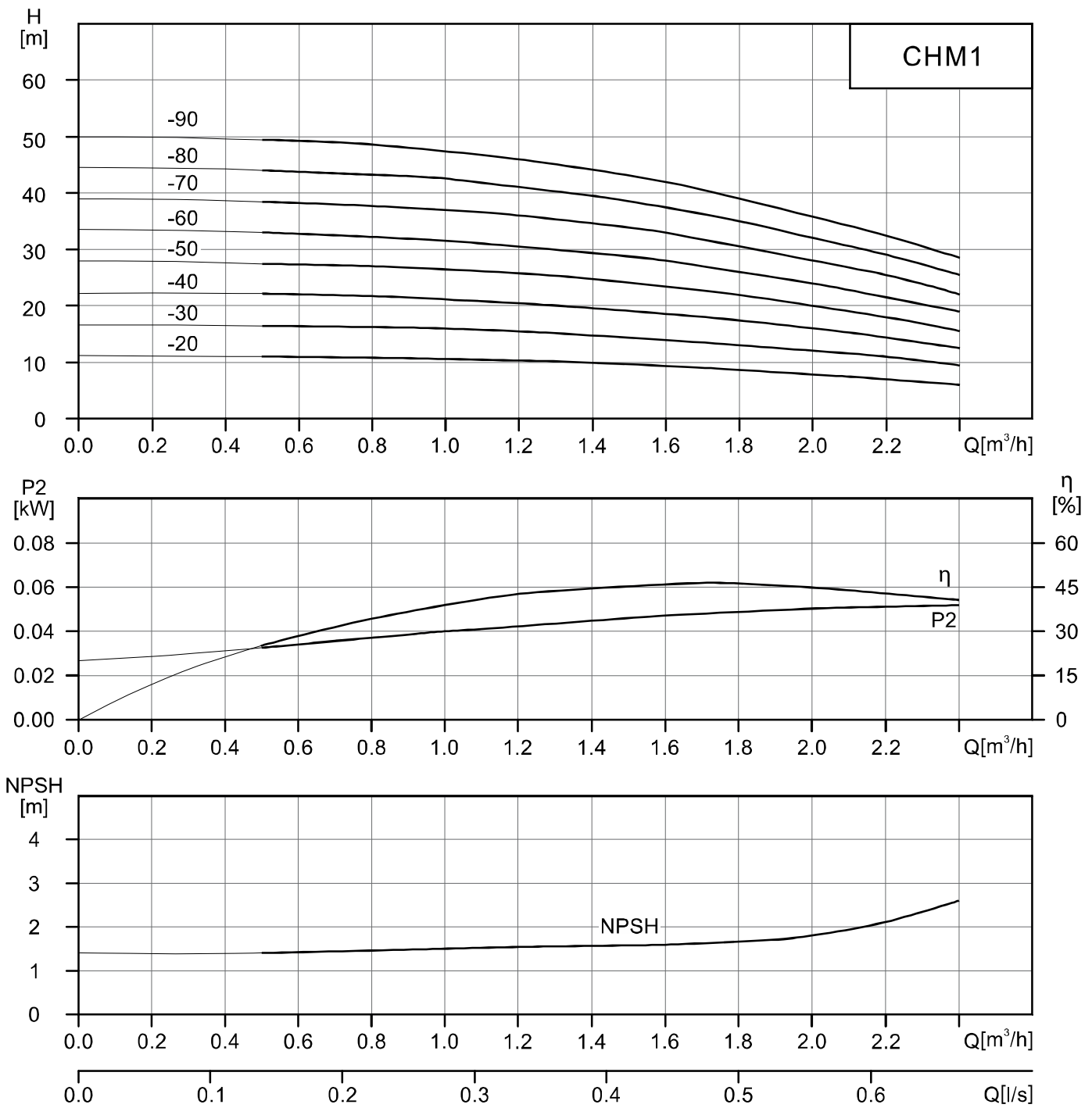
CHM1 性能表
