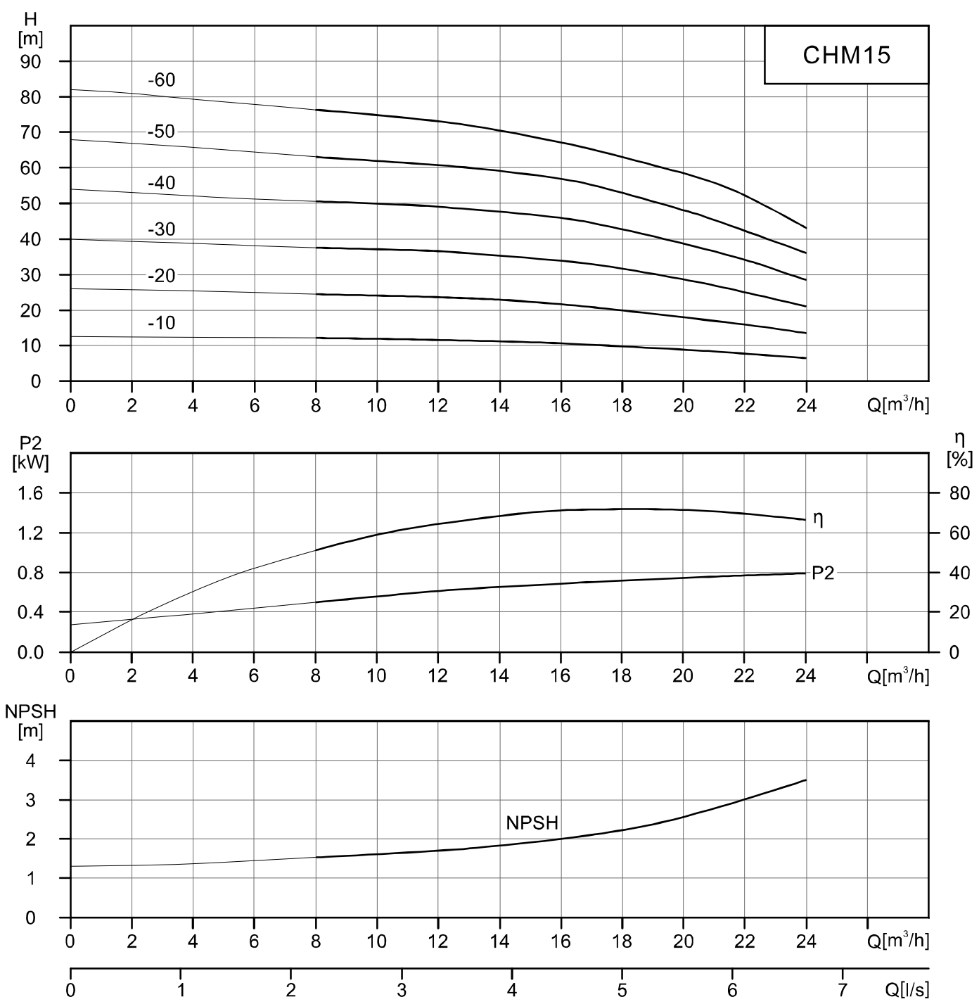
CHM15 性能表
