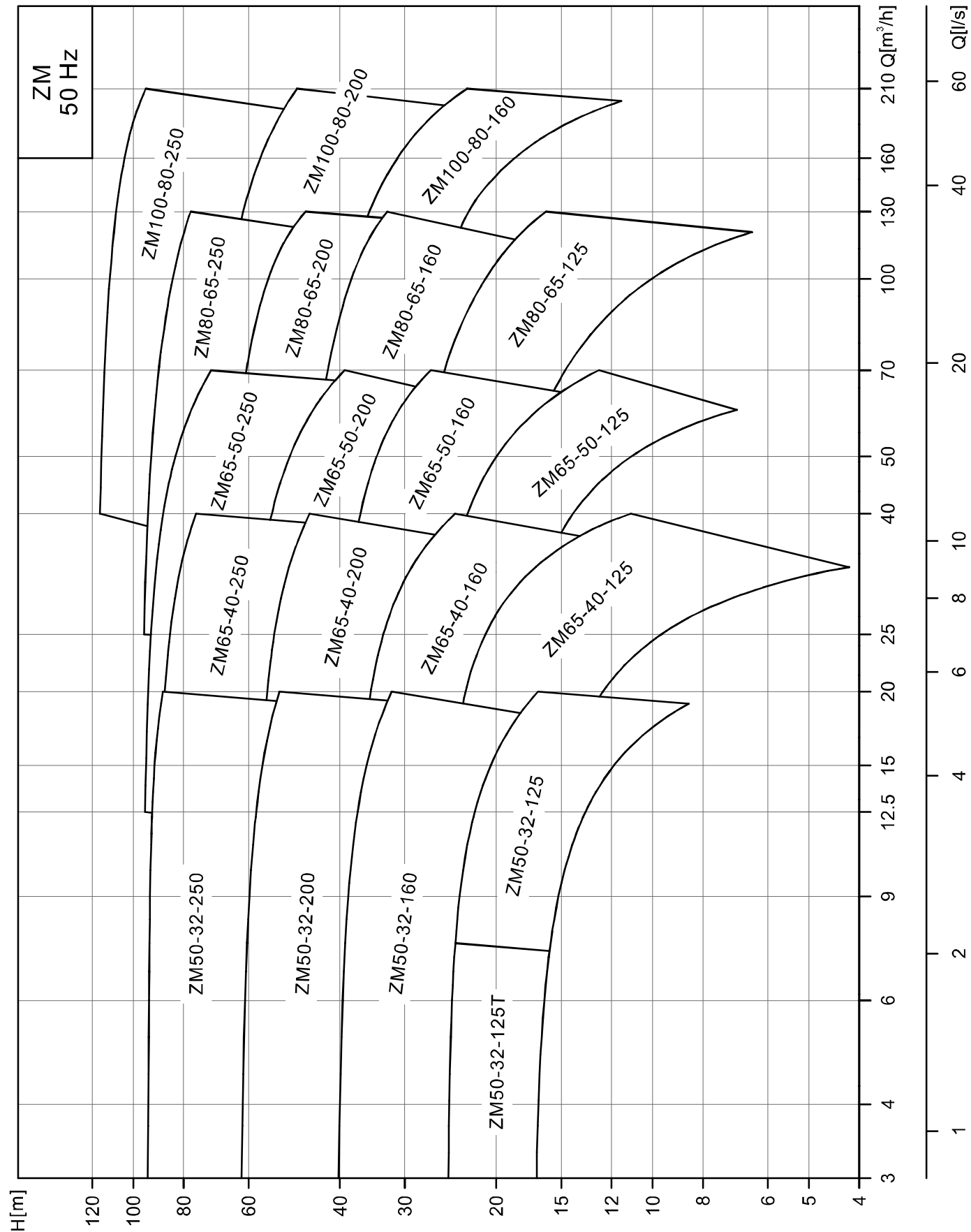
型谱图
