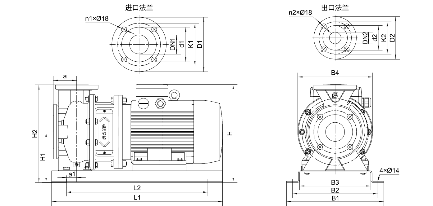
安装尺寸图
