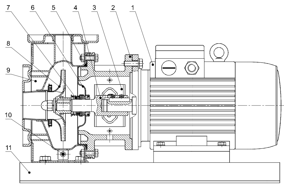
零件材料
