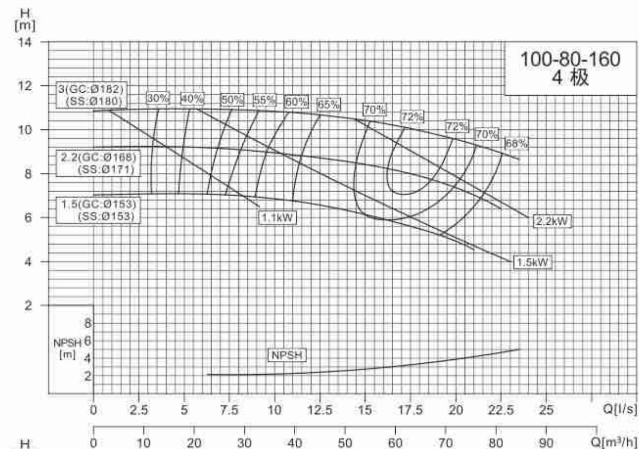
NISO,NIS,NISF100-80-160/125-100-200
