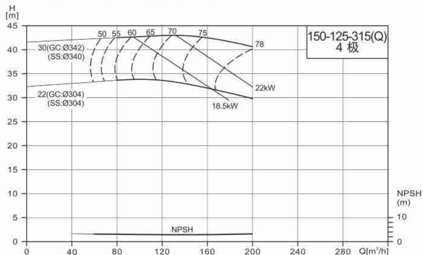
NISO/NIS/NISF150-125-315(Q)/150-125-315G
