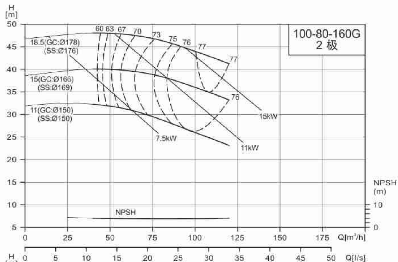
NISO/NIS/NISF100-80-160G/125-100-200(Q)
