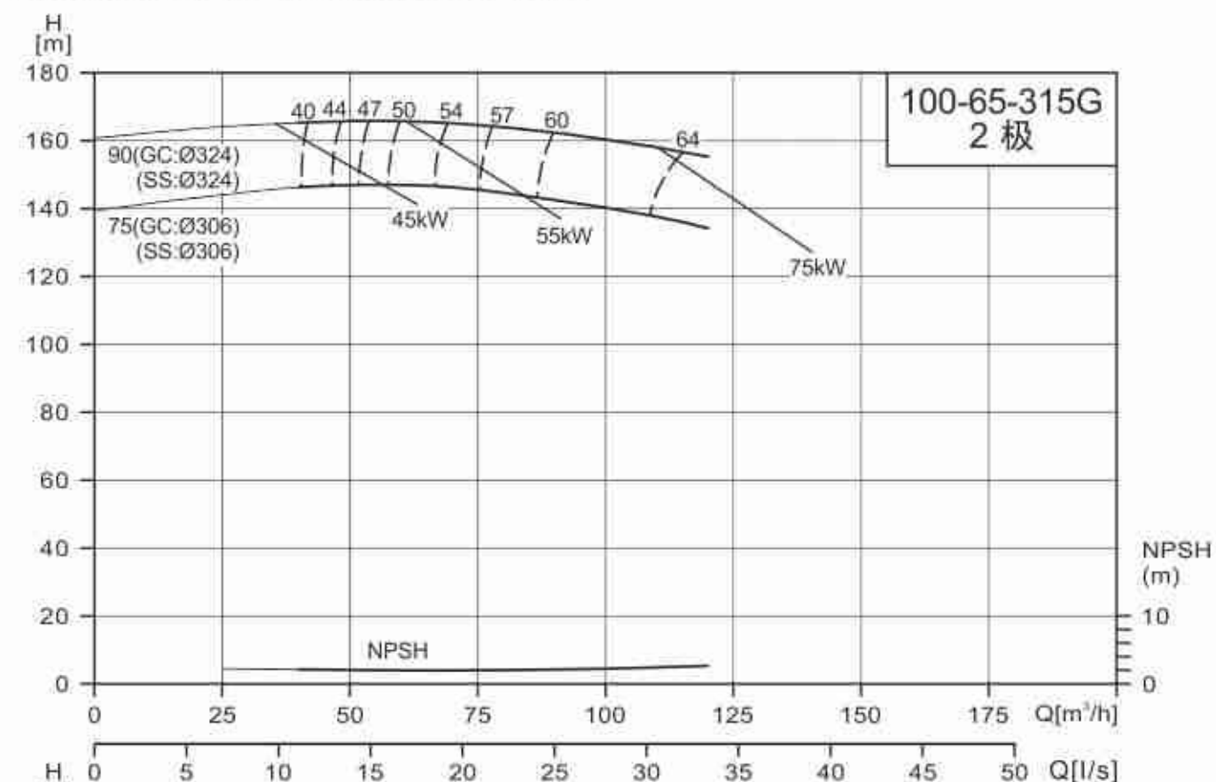
NISO/NIS/NISF100-65-315G/100-80-125G
