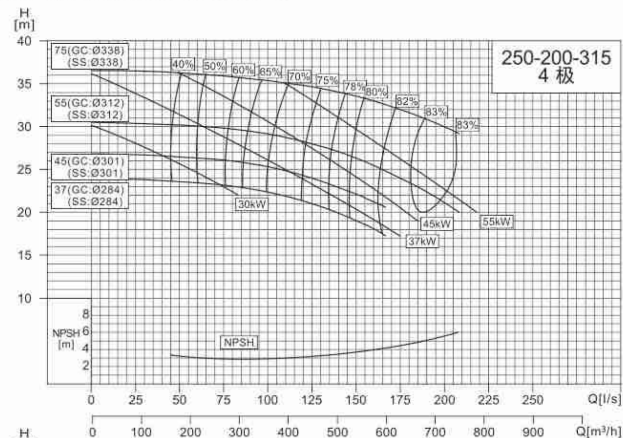
NISO,NIS,NISF250-200-315/250-200-400
