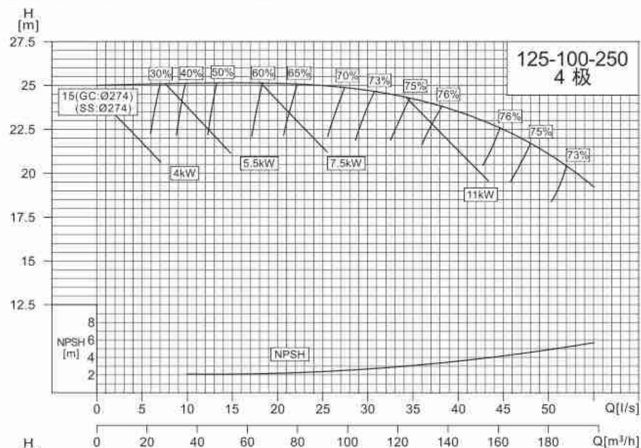
NISO,NIS,NISF125-100-250/125-100-315
