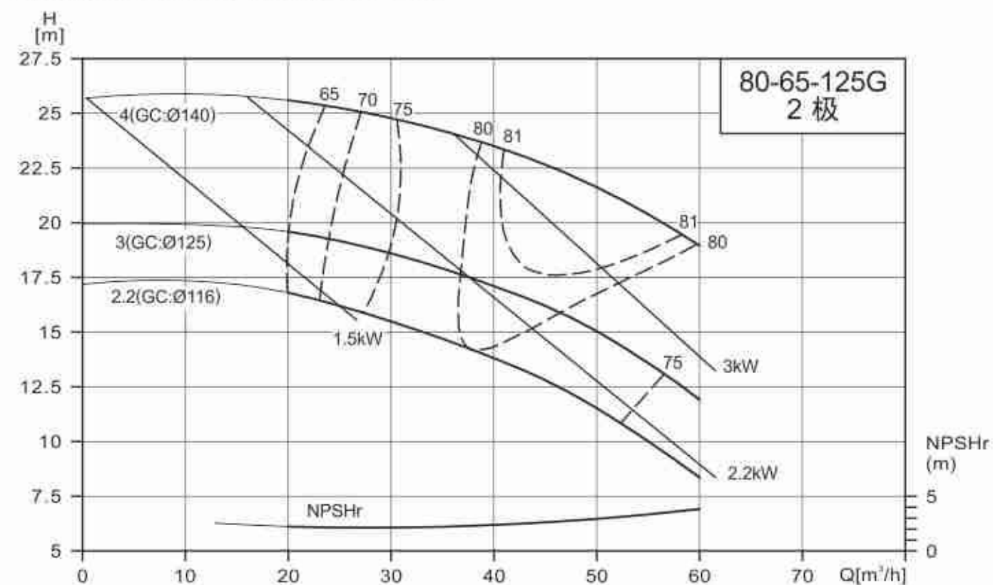
NISO/NIS/NISF80-65-125G/80-65-160G
