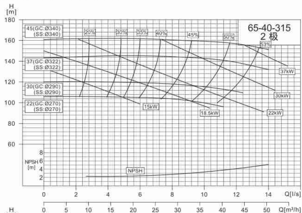
NISO,NIS,NISF65-40-315/65-50-160
