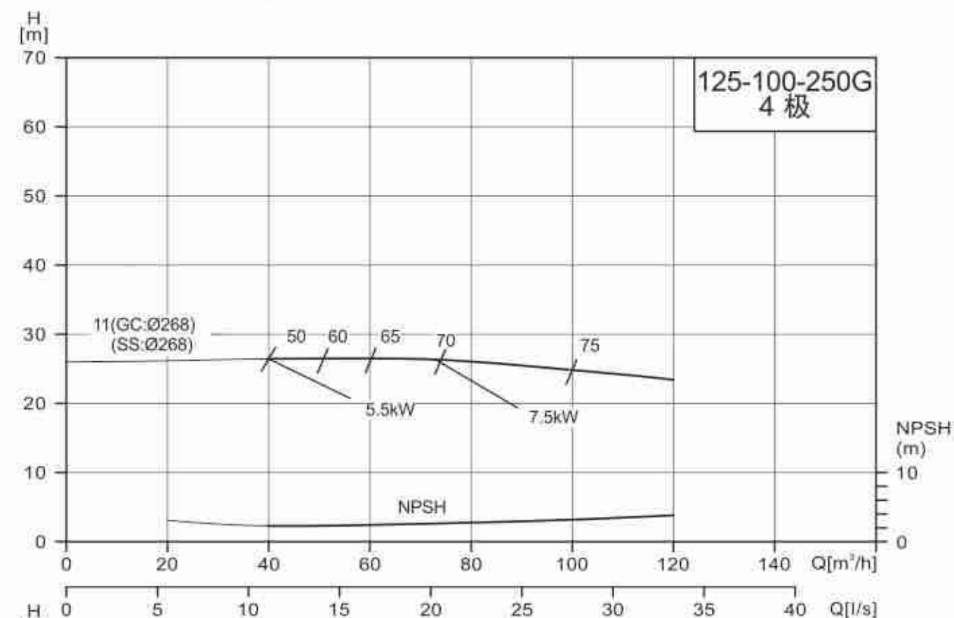
NISO/NIS/NISF125-100-250G/125-100-315G
