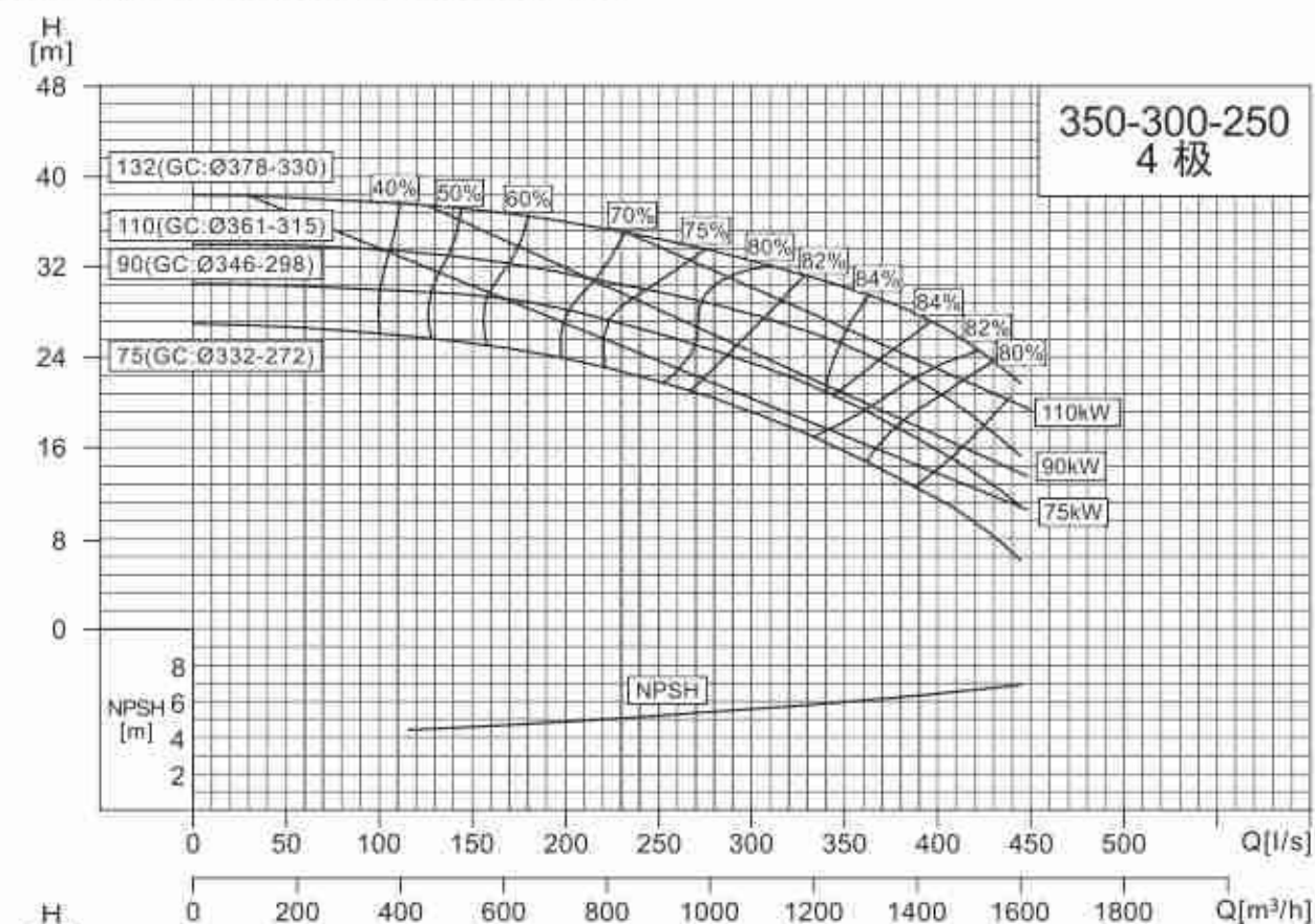
NISO,NIS,NISF350-300-250/350-300-315
