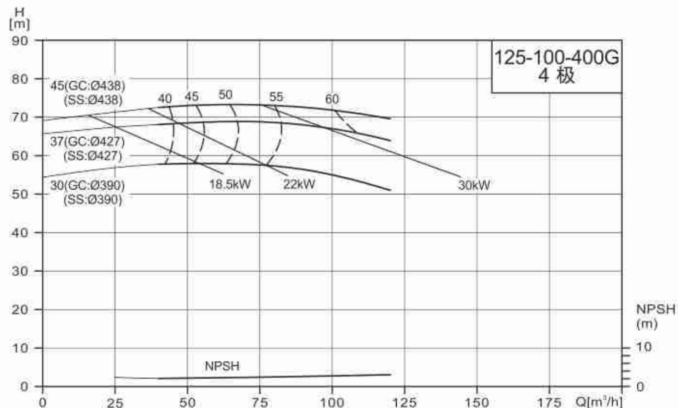
NISO/NIS/NISF125-100-400G/150-125-200(Q)
