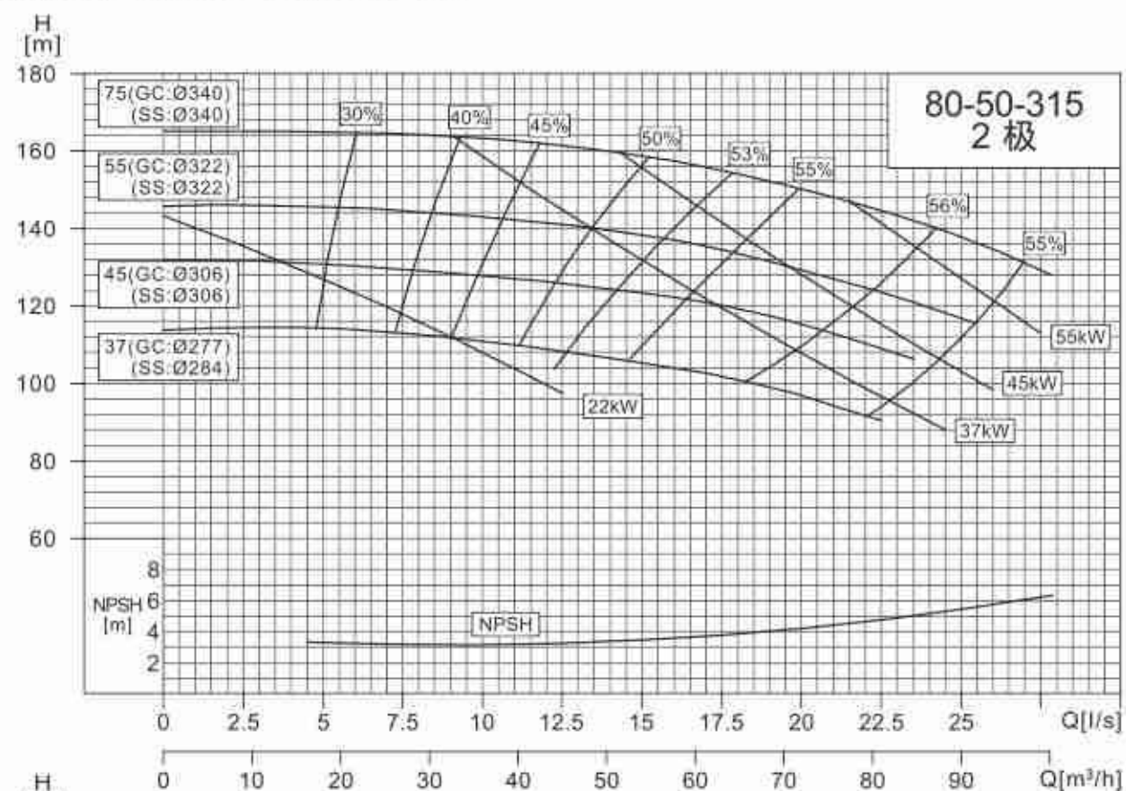
NISO,NIS,NISF80-50-315/80-65-160
