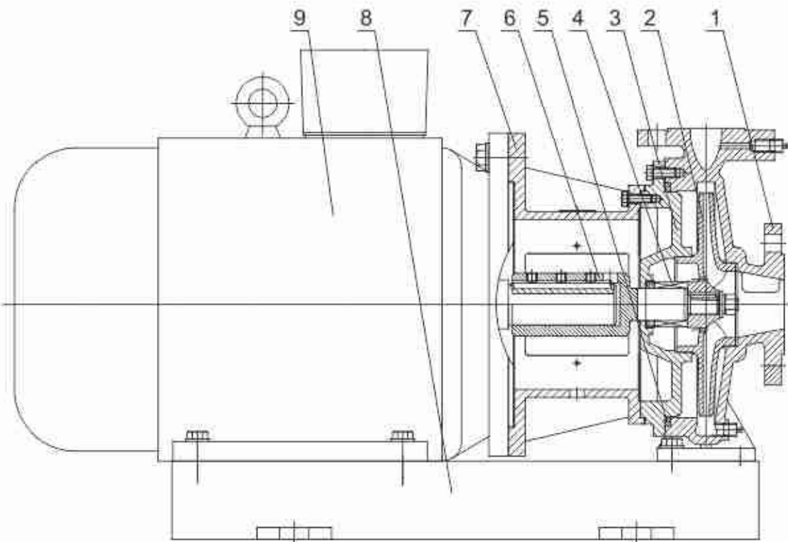
NIS,NISF截面图
