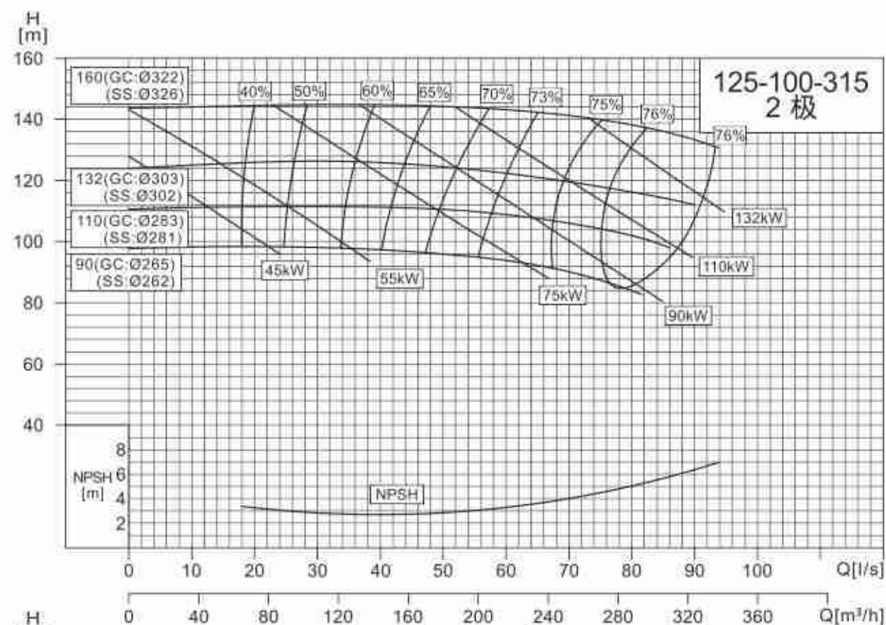
NISO,NIS,NISF125-100-315/50-32-160
