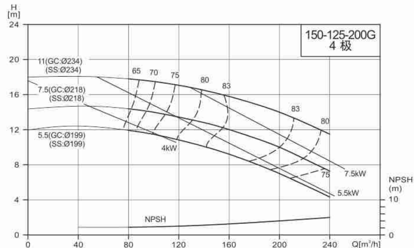
NISO/NIS/NISF150-125-200G/150-125-250G
