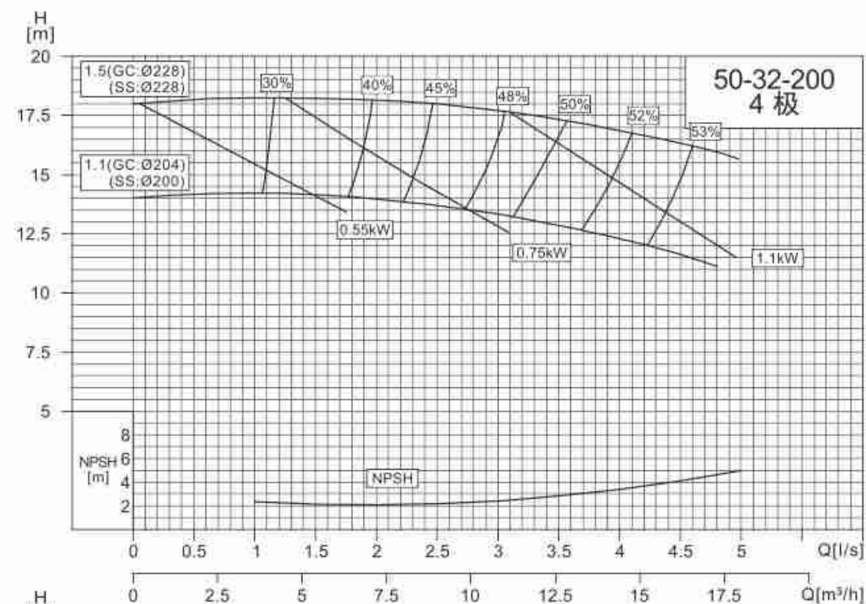
NISO,NIS,NISF50-32-200/65-40-200
