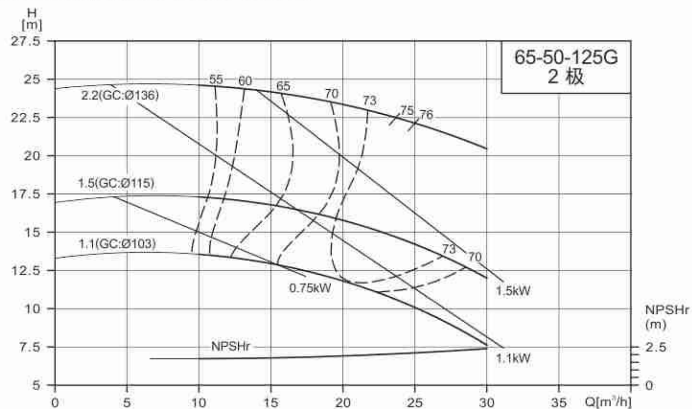
NISO/NIS/NISF65-50-125G/65-50-160G
