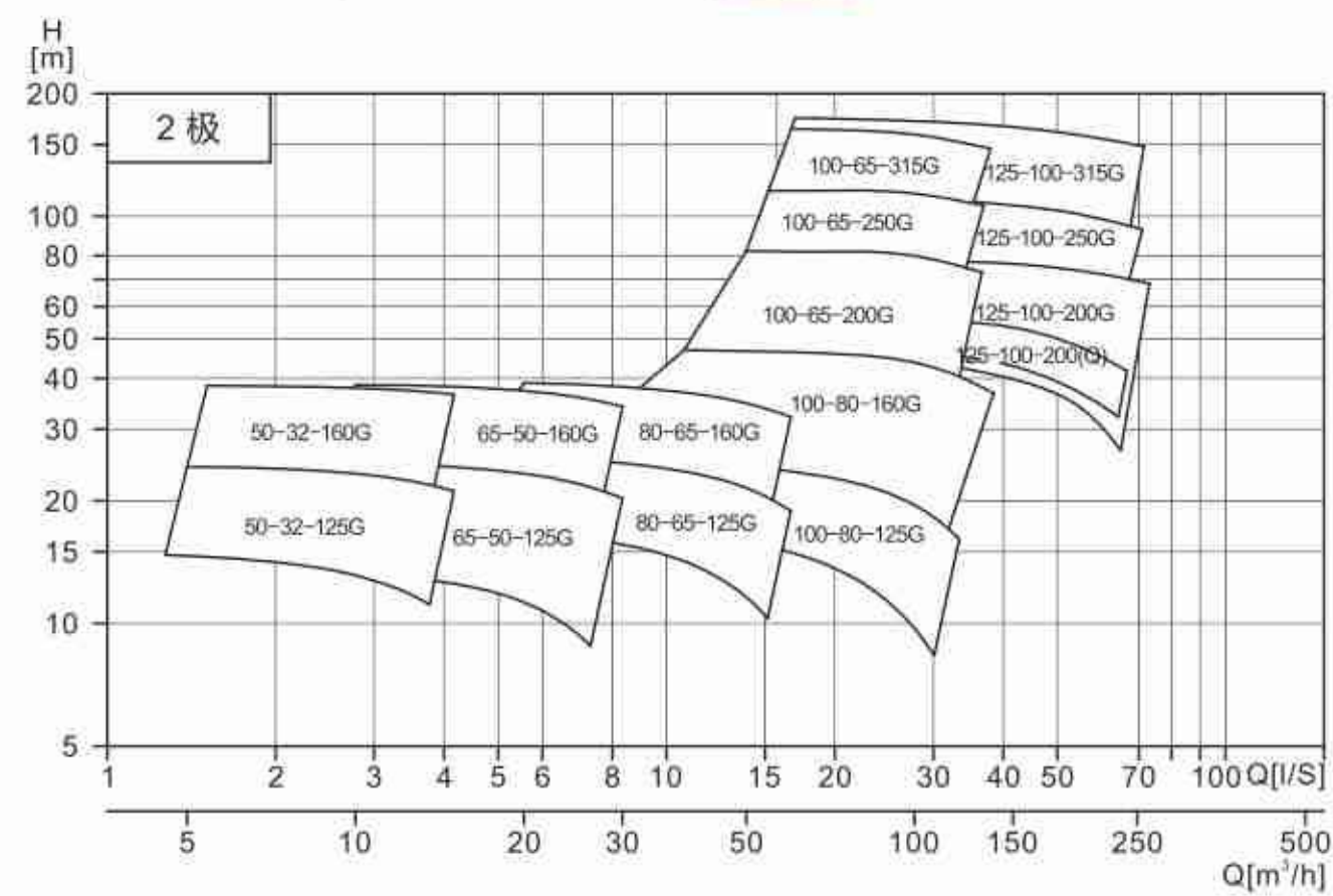
NISO/NIS/NISF*G,NISO/NIS/NISF*(Q)型谱图
