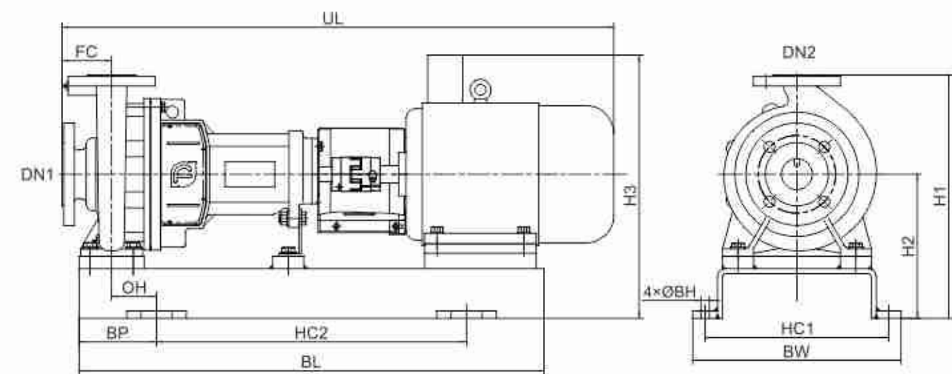
NISO*G,NISO*(Q)泵组外形尺寸表
