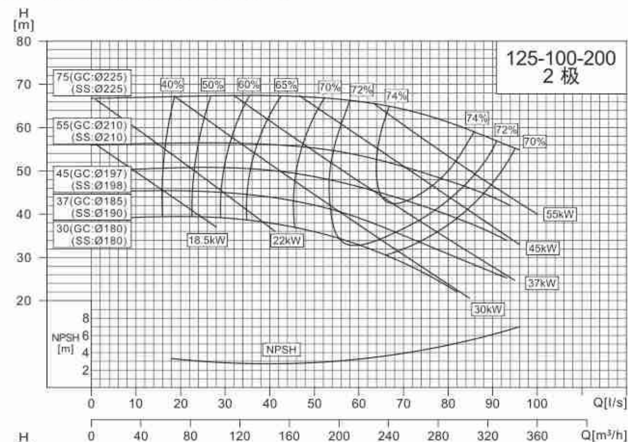
NISO,NIS,NISF125-100-200/125-100-250
