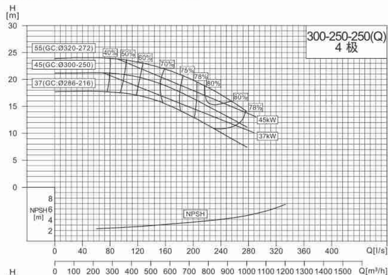
NISO,NIS,NISF300-250-250(Q)/300-250-250
