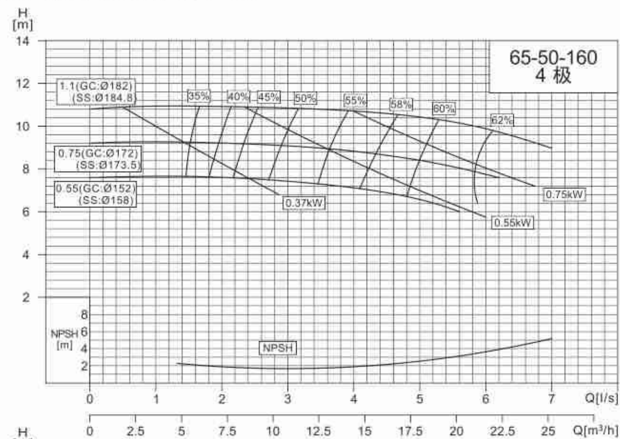
NISO,NIS,NISF65-50-160/80-50-200
