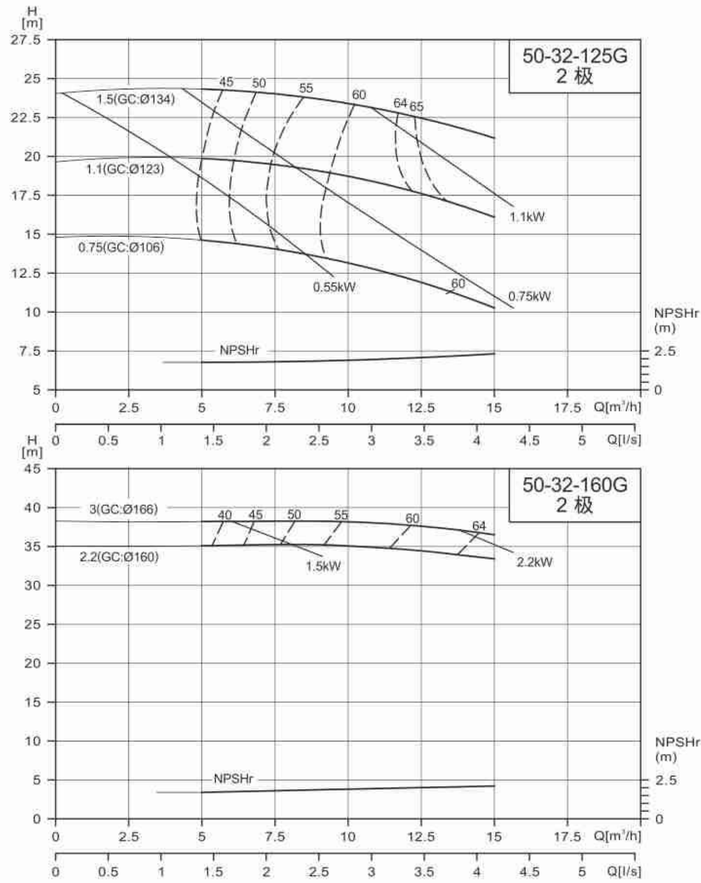
NISO/NIS/NISF50-32-125G/50-32-160G
