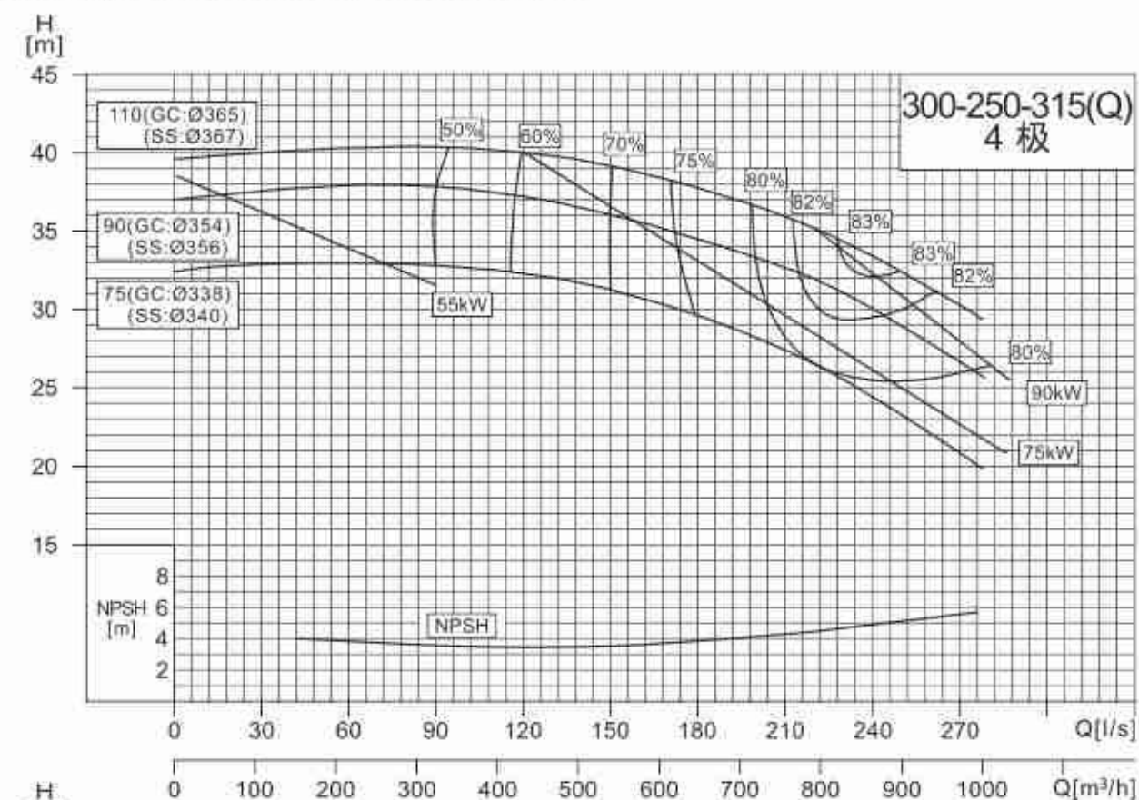
NISO,NIS,NISF300-250-315(Q)/300-250-315
