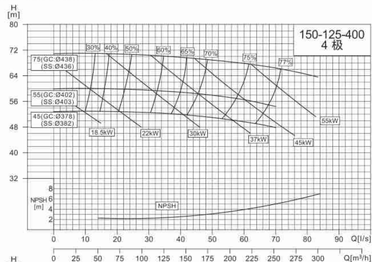
NISO,NIS,NISF150-125-400/200-150-315
