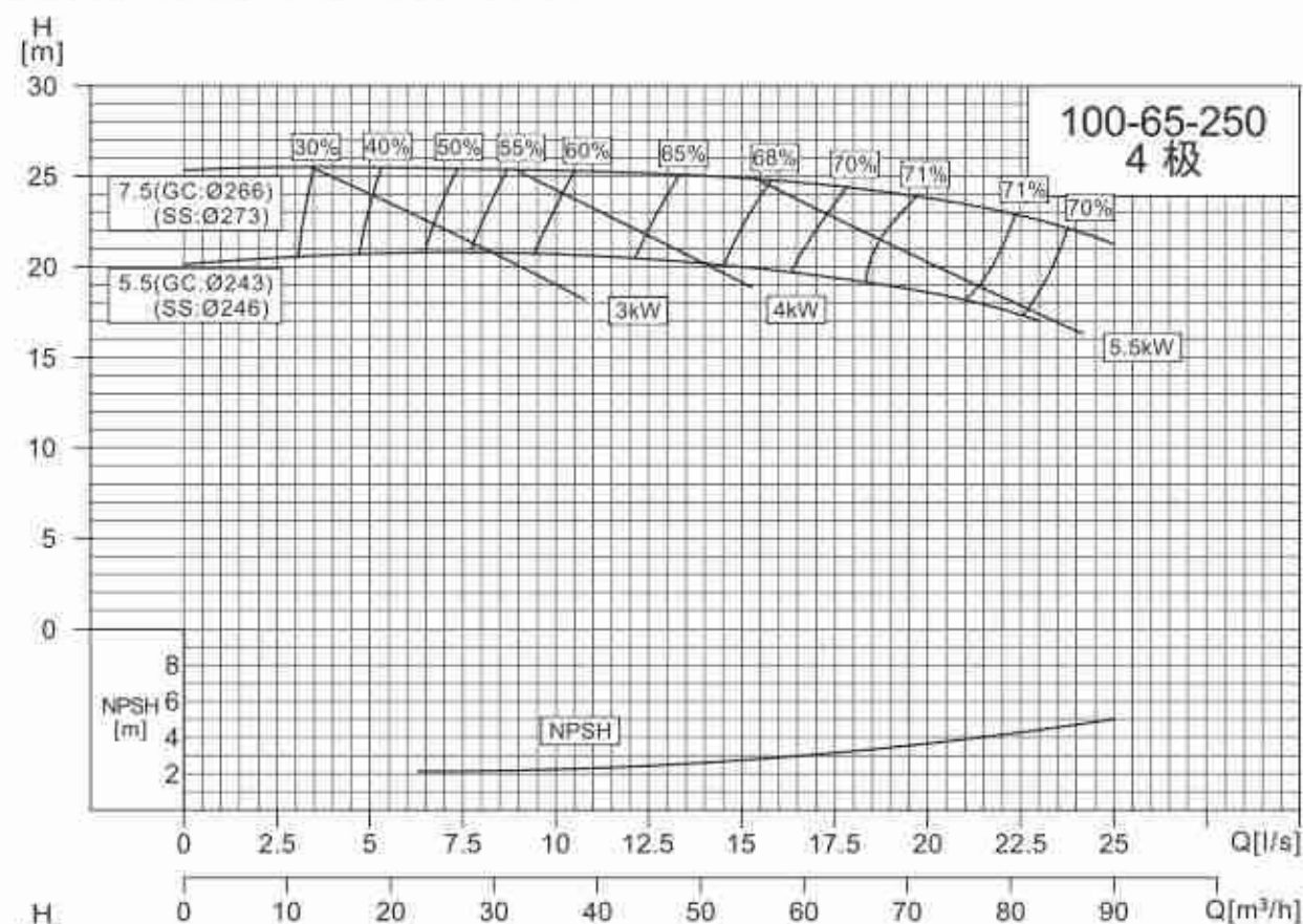
NISO,NIS,NISF100-65-250/100-65-315
