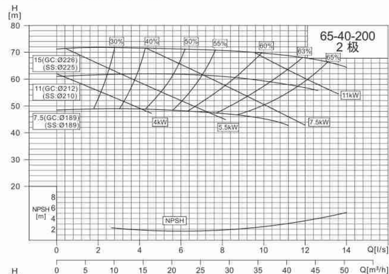
NISO,NIS,NISF65-40-200/65-40-250
