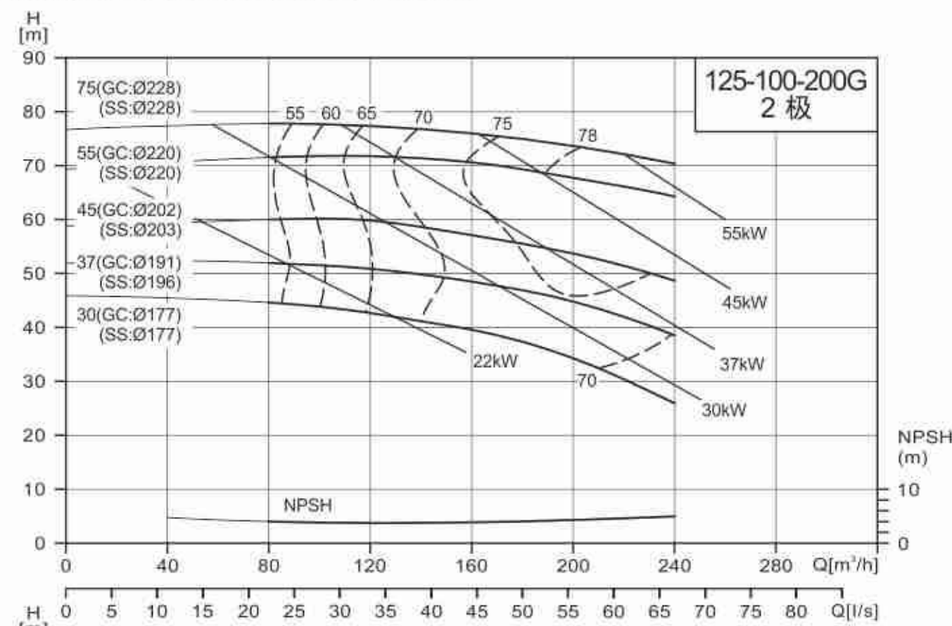
NISO/NIS/NISF125-100-200G/125-100-250G
