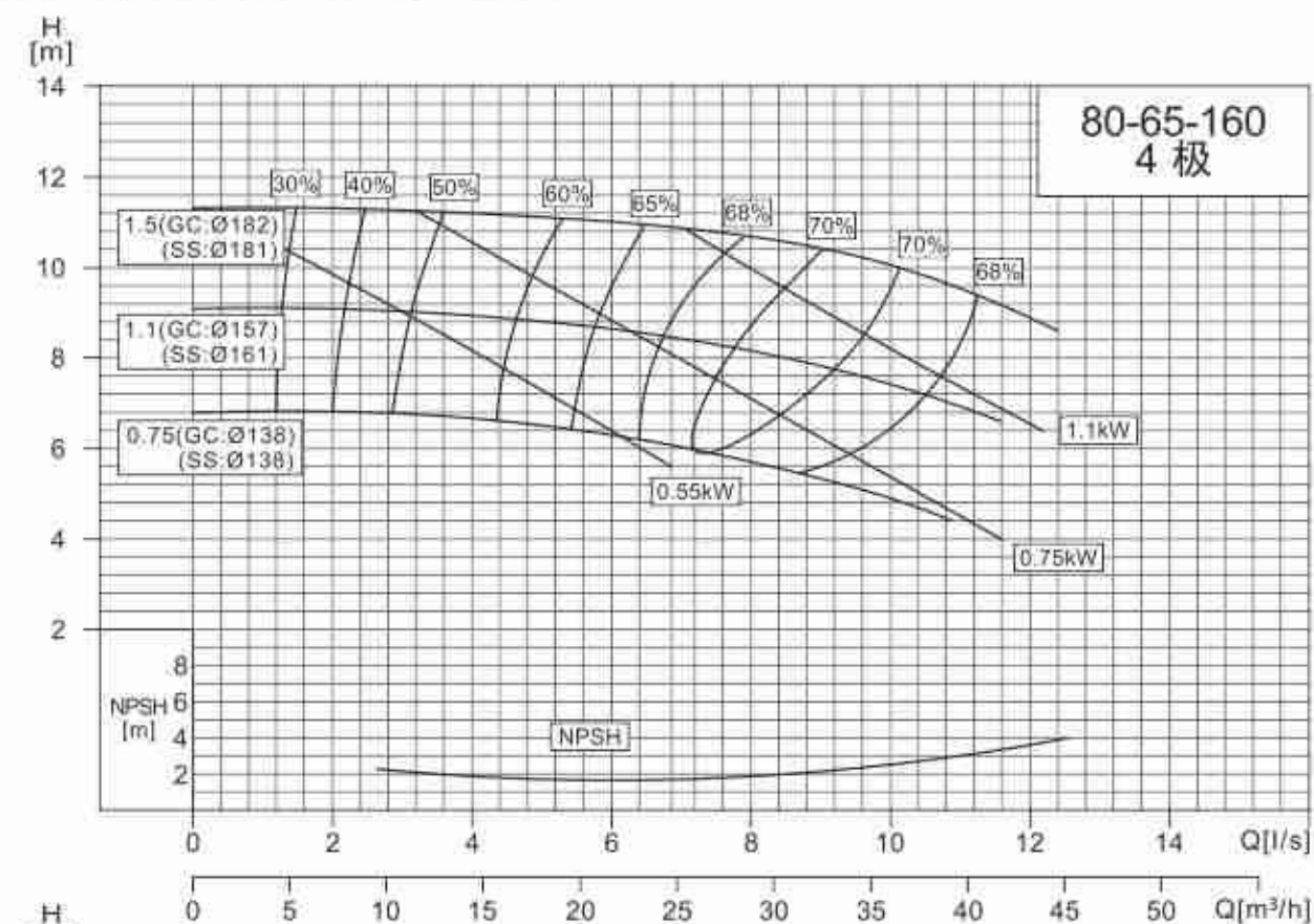
NISO,NIS,NISF80-65-160/100-65-200
