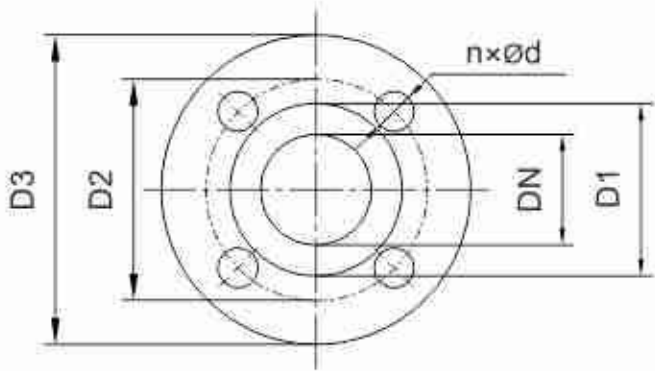
NIS/NISF*G,NIS/NISF*(Q)法兰
