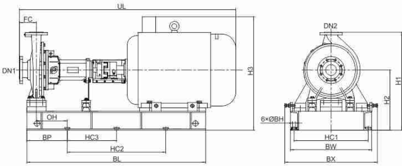
NISO*G,NISO*(Q)泵组外形尺寸图(槽钢底座结构)
