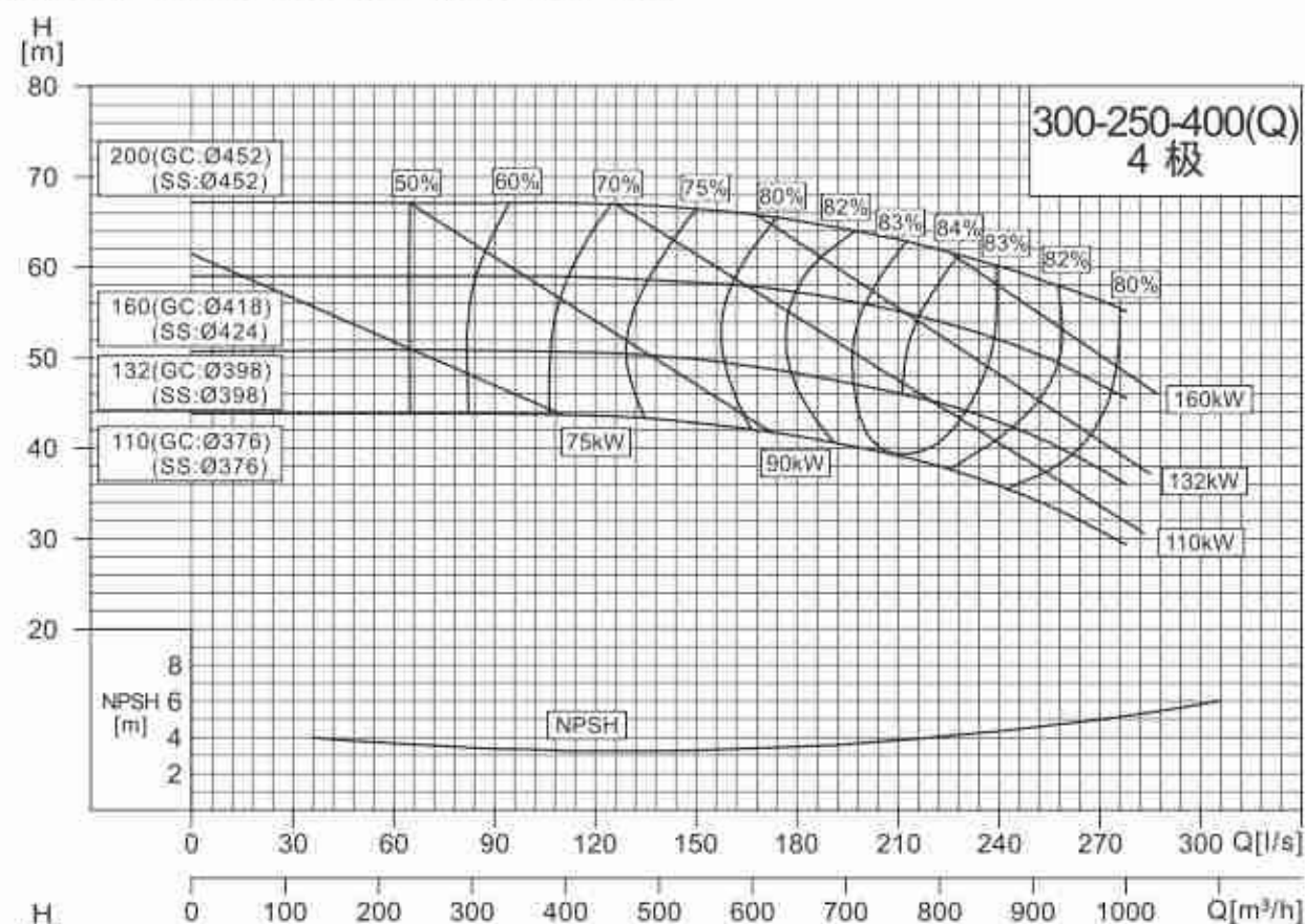
NISO,NIS,NISF300-250-400(Q)/300-250-400
