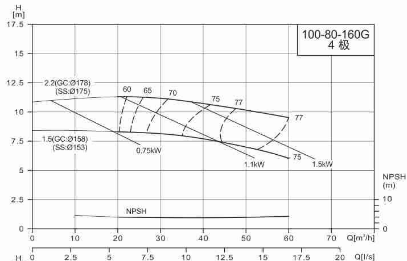
NISO/NIS/NISF100-80-160G/125-100-200G
