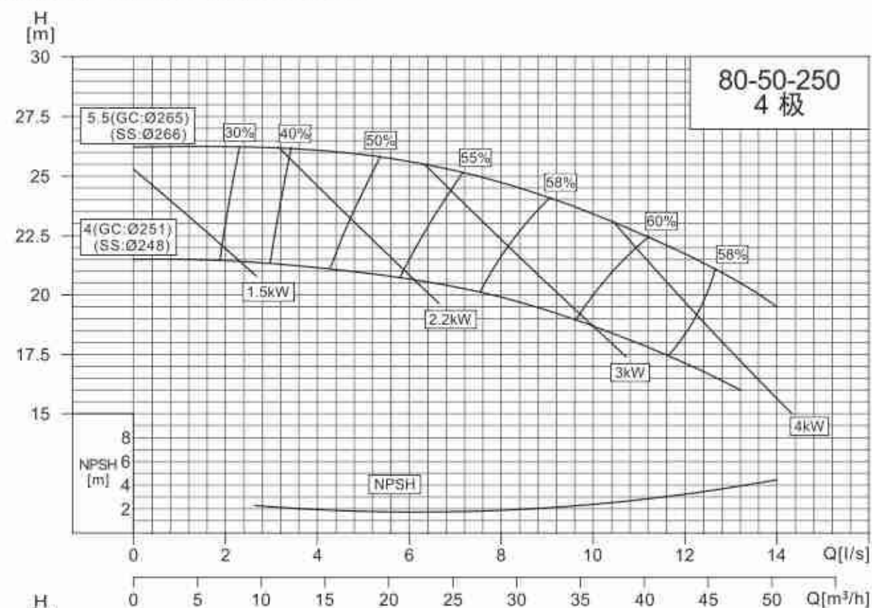
NISO,NIS,NISF80-50-250/80-50-315
