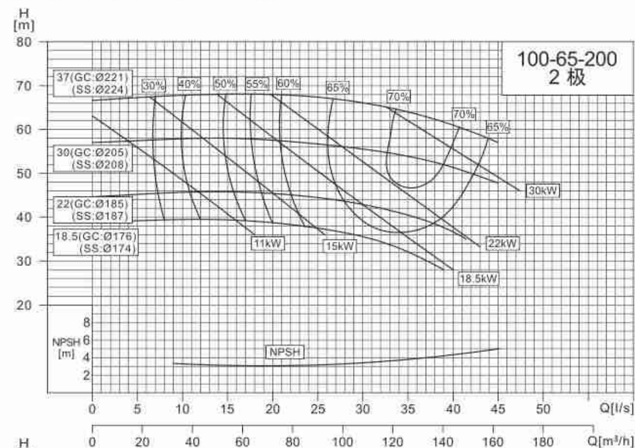
NISO,NIS,NISF100-65-200/100-65-250
