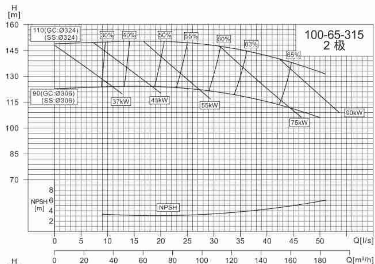
NISO,NIS,NISF100-65-315/100-80-160
