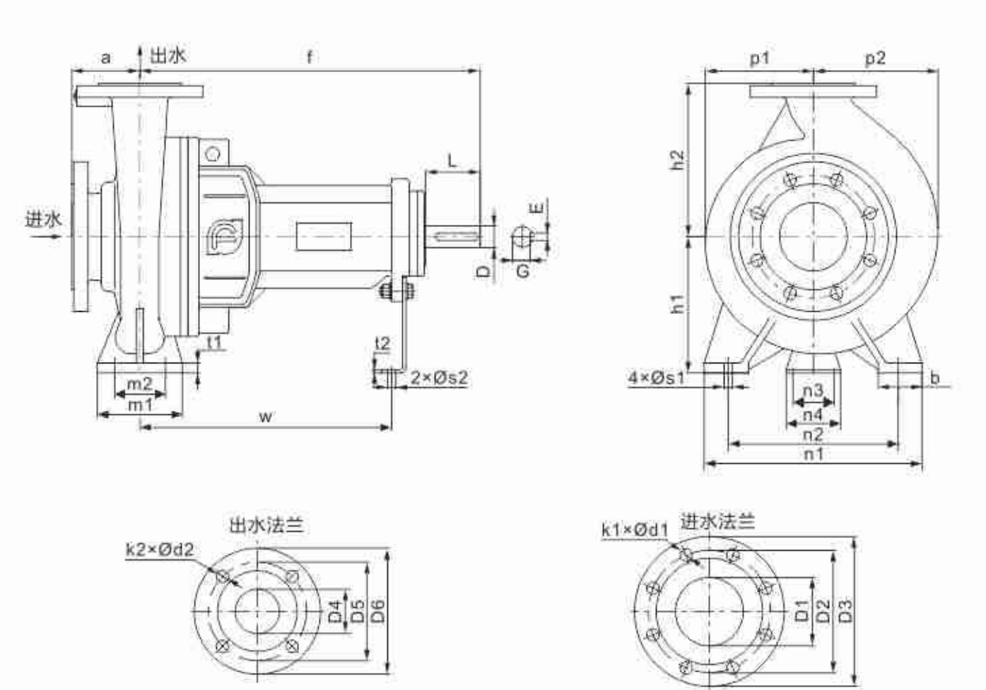
NISO*G,NISO*(Q)泵外形尺寸图
