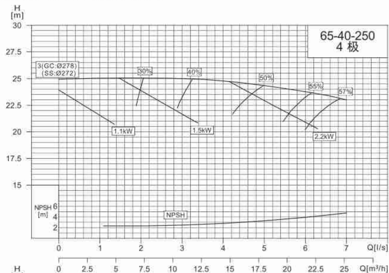
NISO,NIS,NISF65-40-250/65-40-315
