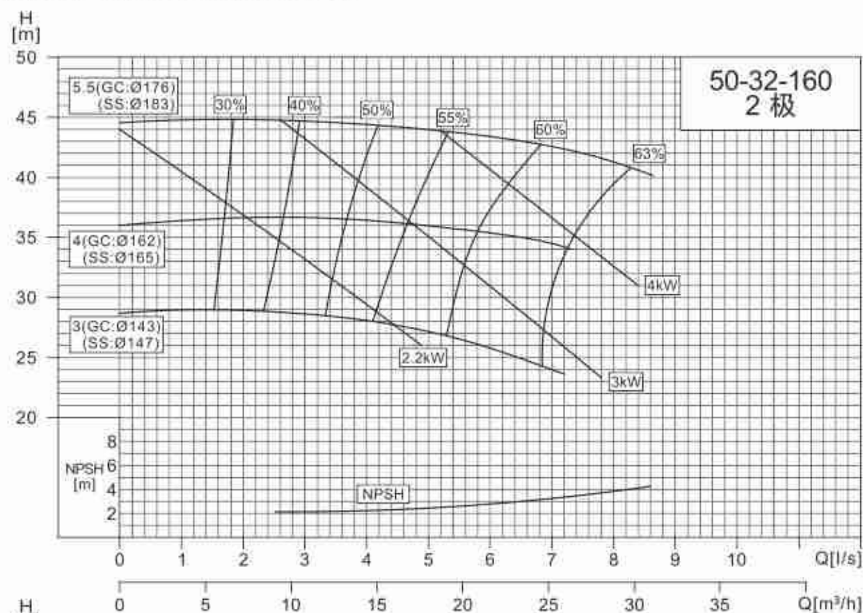
NISO,NIS,NISF50-32-160/50-32-200
