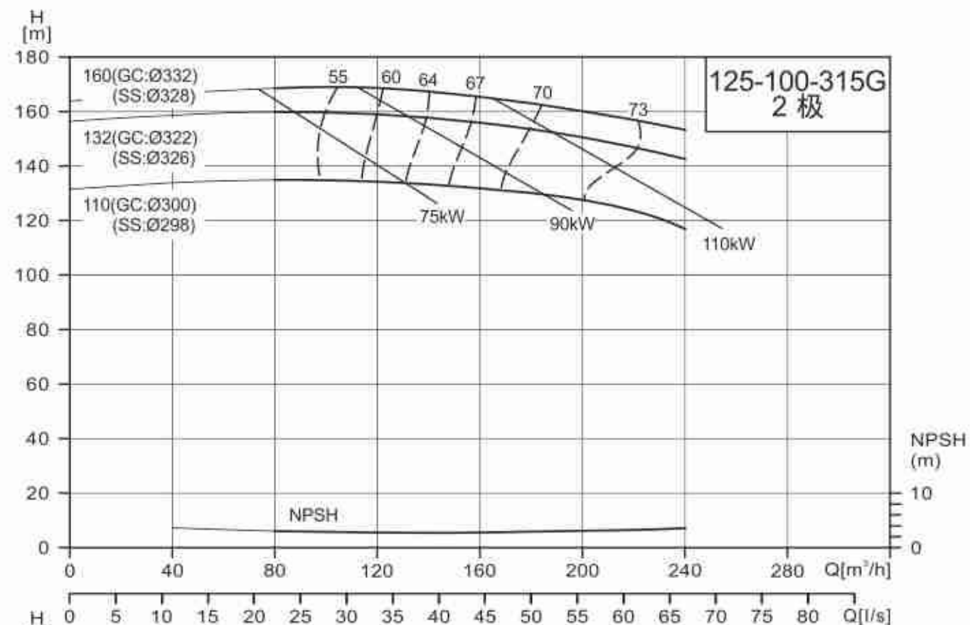
NISO/NIS/NISF125-100-315G/100-65-200G
