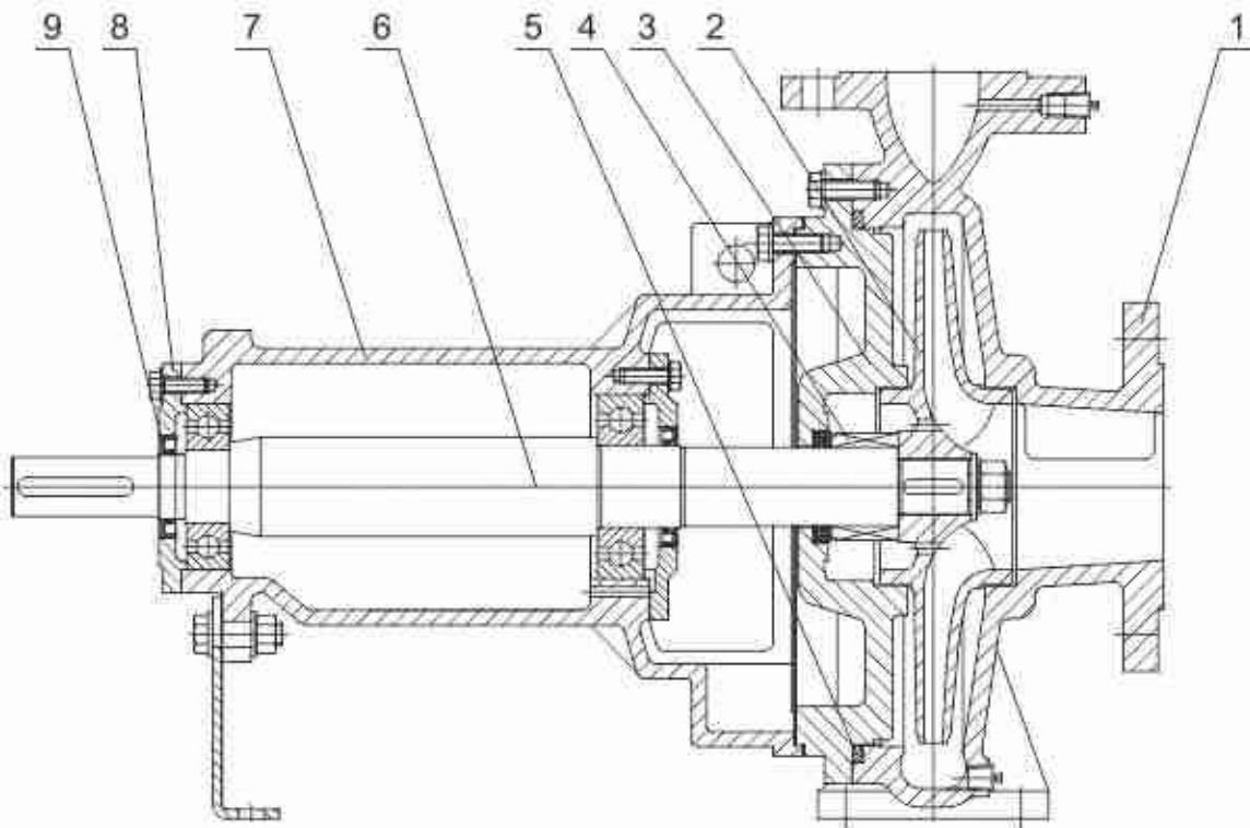
NISO截面图
