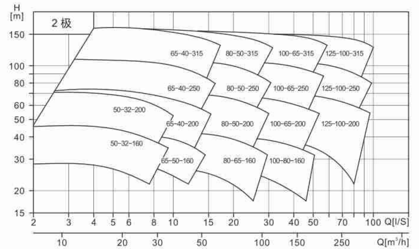
NISO,NIS,NISF型谱图
