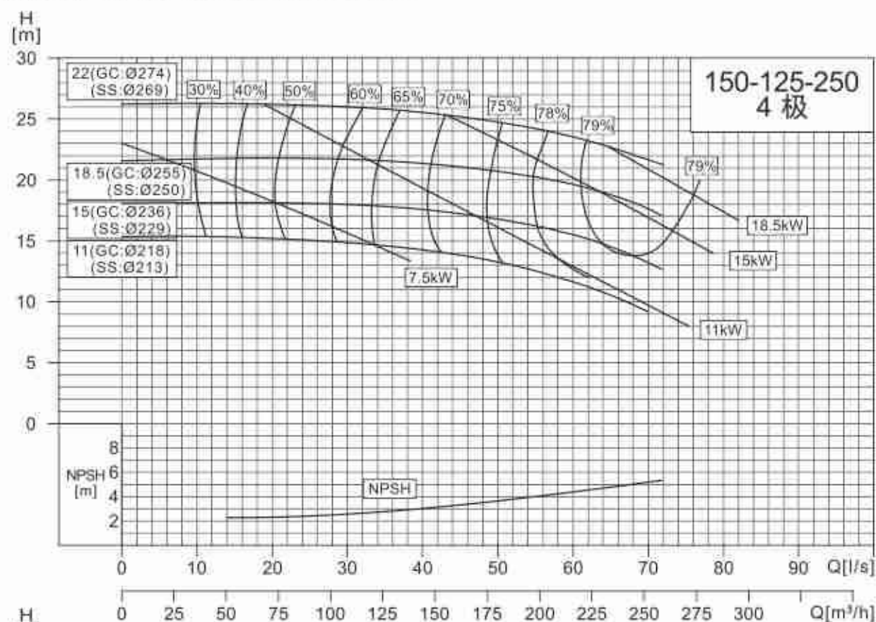
NISO,NIS,NISF150-125-250/150-125-315
