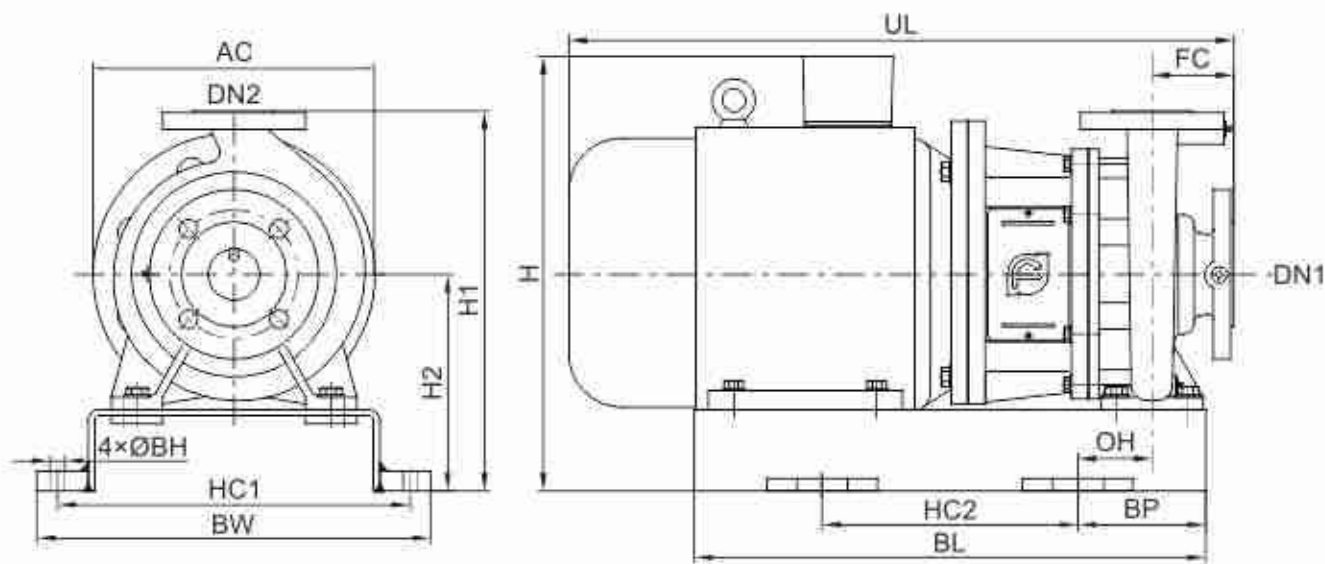
NIS,NISF泵外形尺寸图
