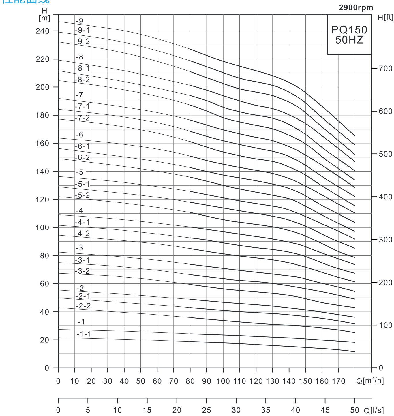
性能曲线
