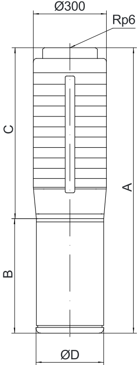
PQ200安装尺寸图
