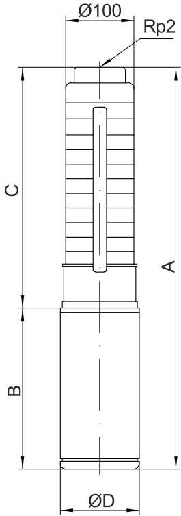
PQ8安装尺寸图
