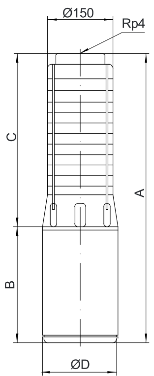
PQ60安装尺寸图
