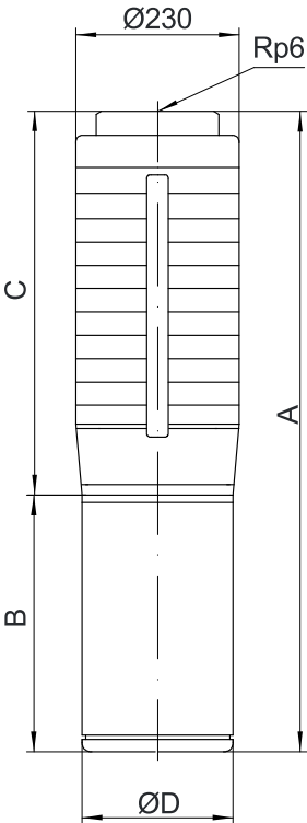
PQ150安装尺寸图
