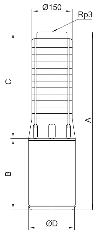
PQ42安装尺寸图
