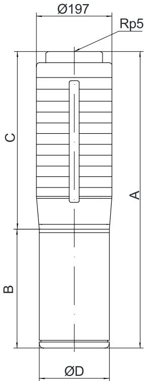
PQ95安装尺寸图
