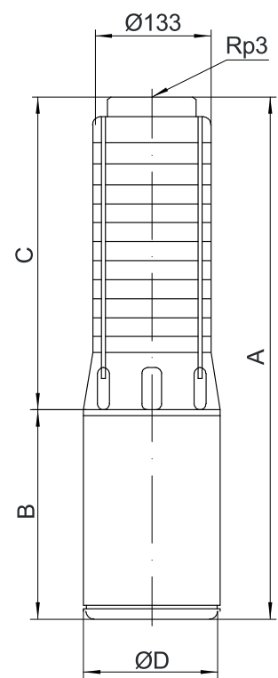
PQ30安装尺寸图
