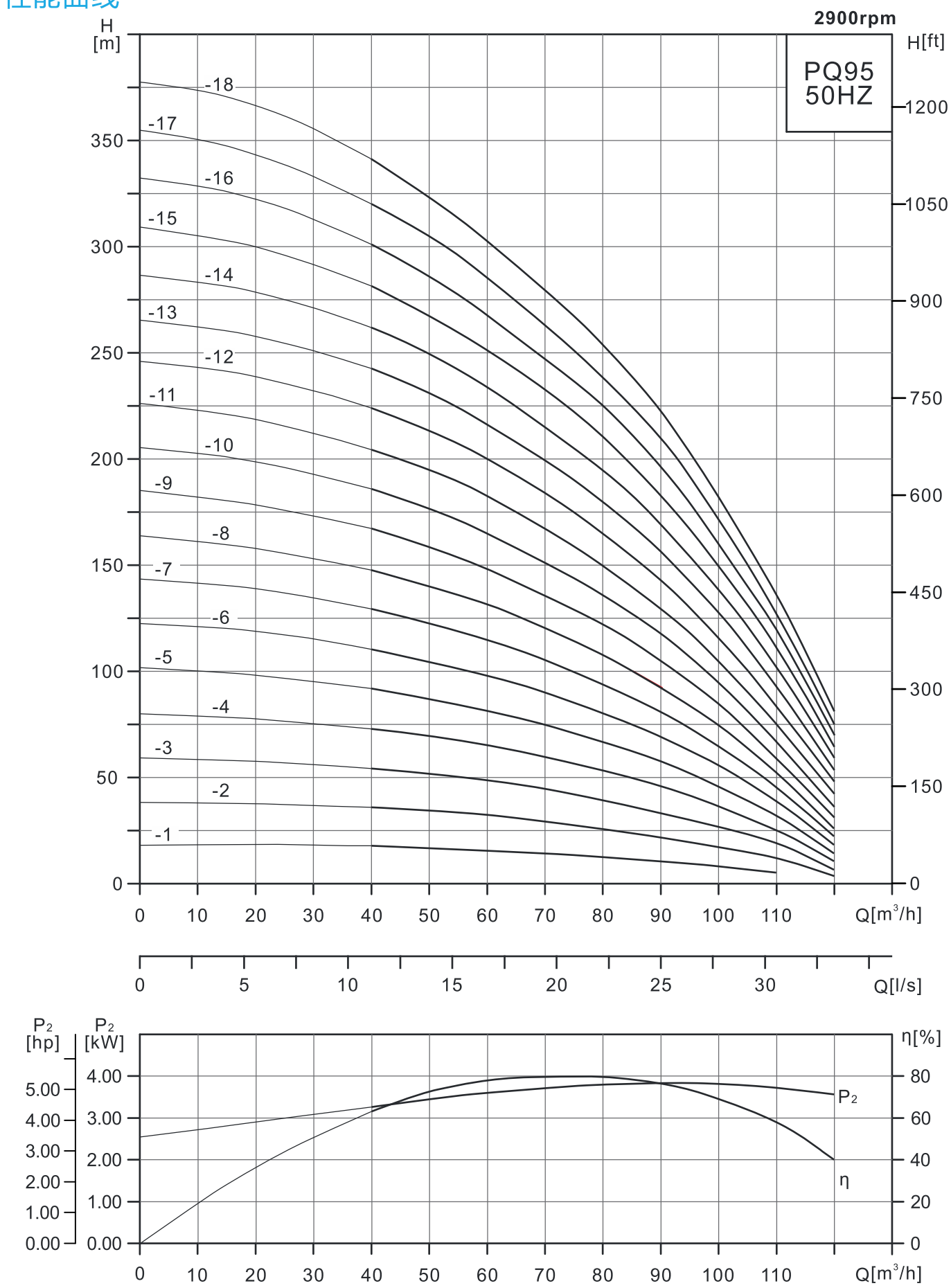
性能曲线
