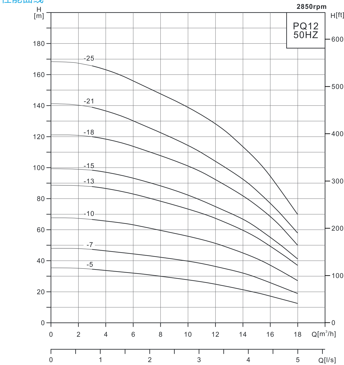
性能曲线
