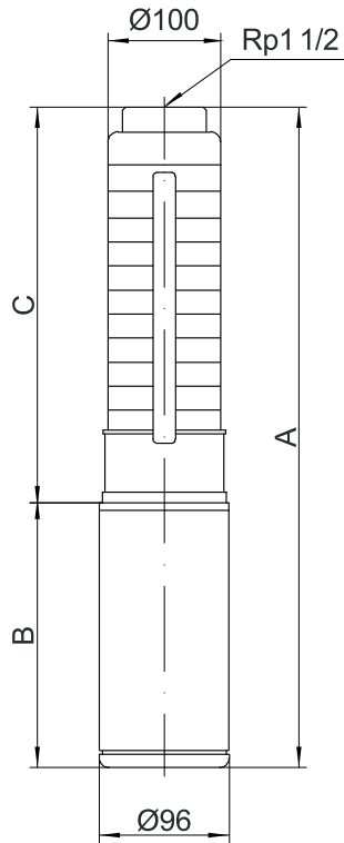
PQ5安装尺寸图
