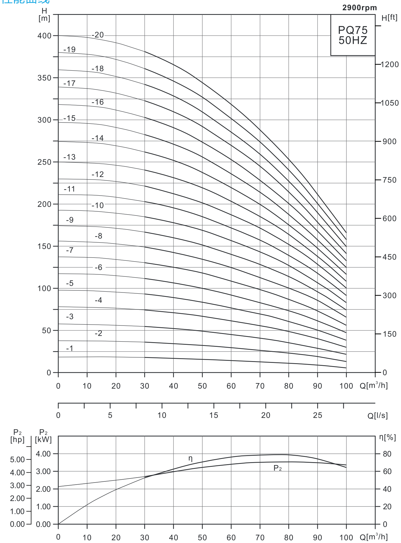
性能曲线
