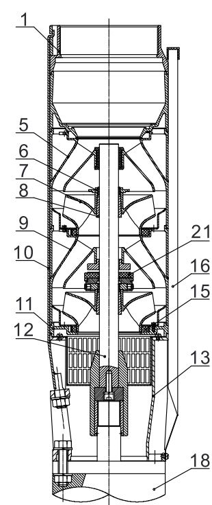
PQ150截面图
