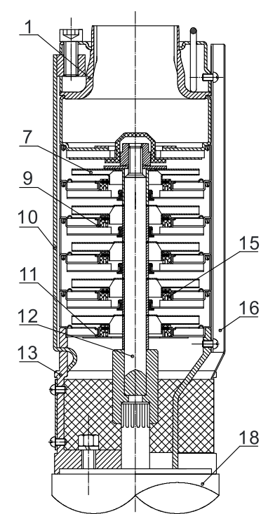
PQ5截面图
