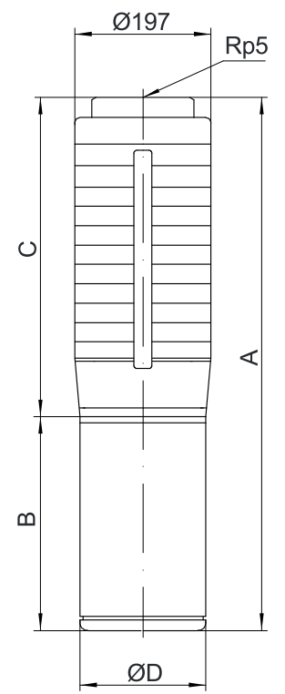
PQ75安装尺寸图
