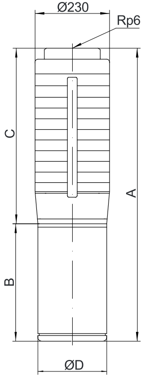
PQ120安装尺寸图
