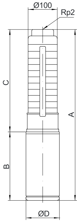
PQ12安装尺寸图
